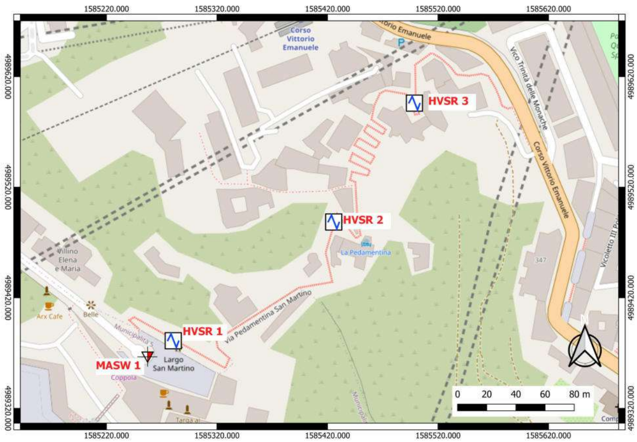
Fig. 36 – Ubicazione Indagini
