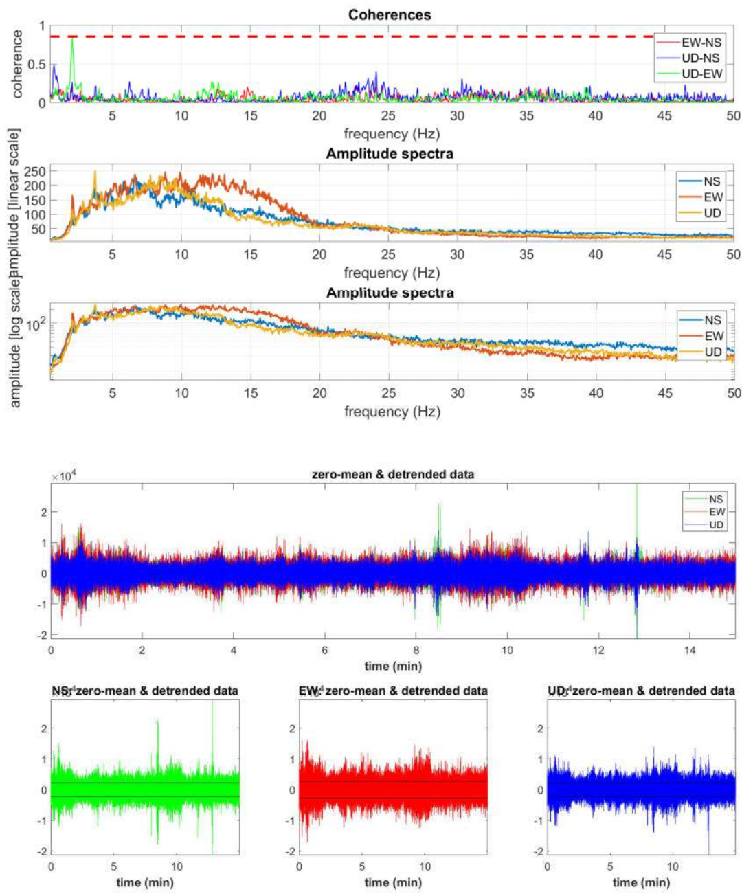
Fig. 20 - Acquisizione dati HVSR
