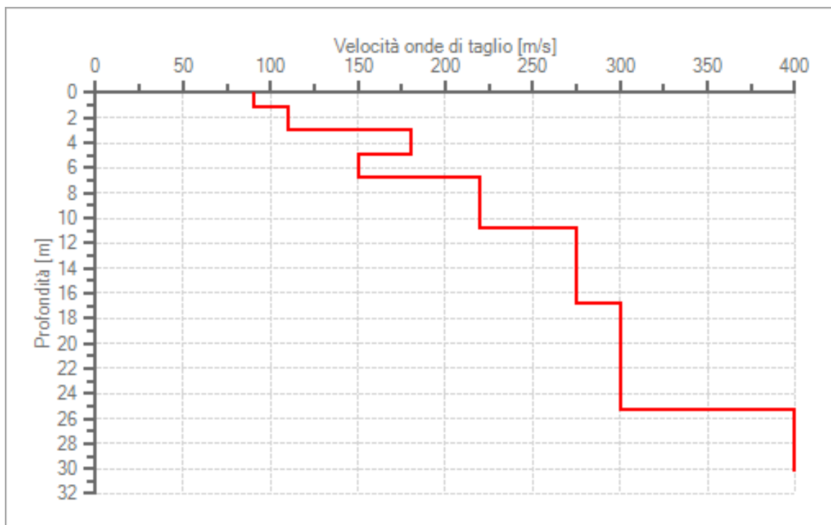
Fig. 8 - Profilo delle velocità delle onde di taglio.
