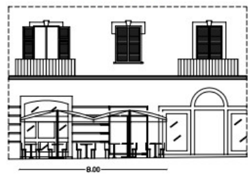
STATO DI PROGETTO Prospetto - Scala 1:100
