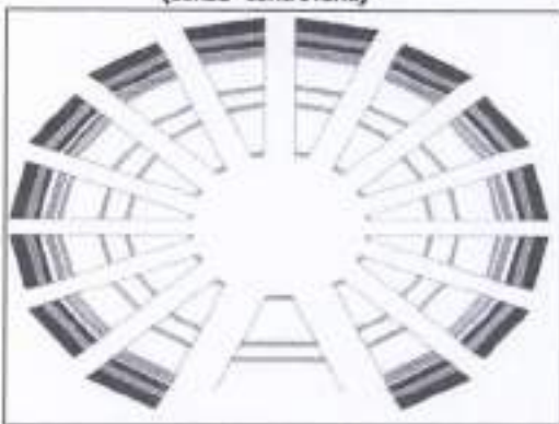
SCHEMA DI MONTAGGIO A SPICCHI VISTO DALL'ALTO (senza controventi)
