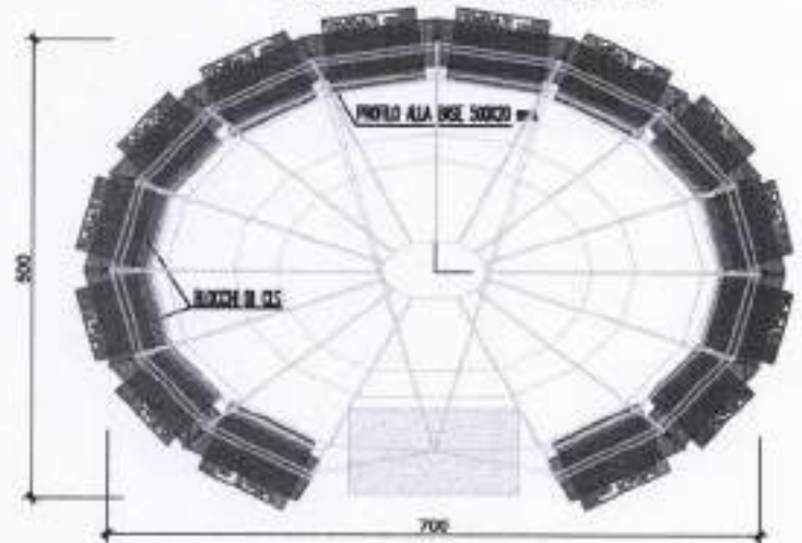
PIANTA ALLA BASE 1:50
