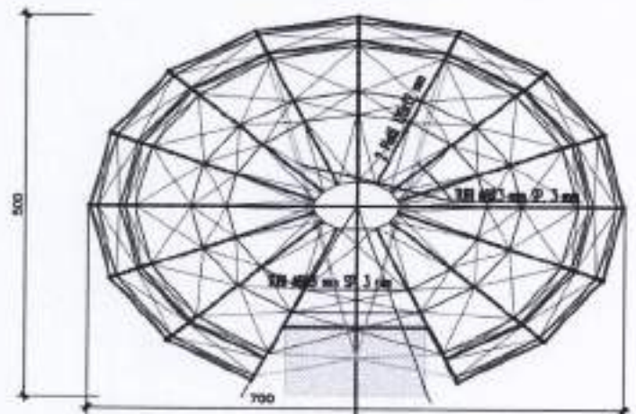
PIANTA ALLA BASE 1:50
