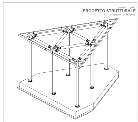
Figura 15 Modellazione strutturale
