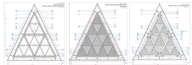
Figura 17 Coperture
