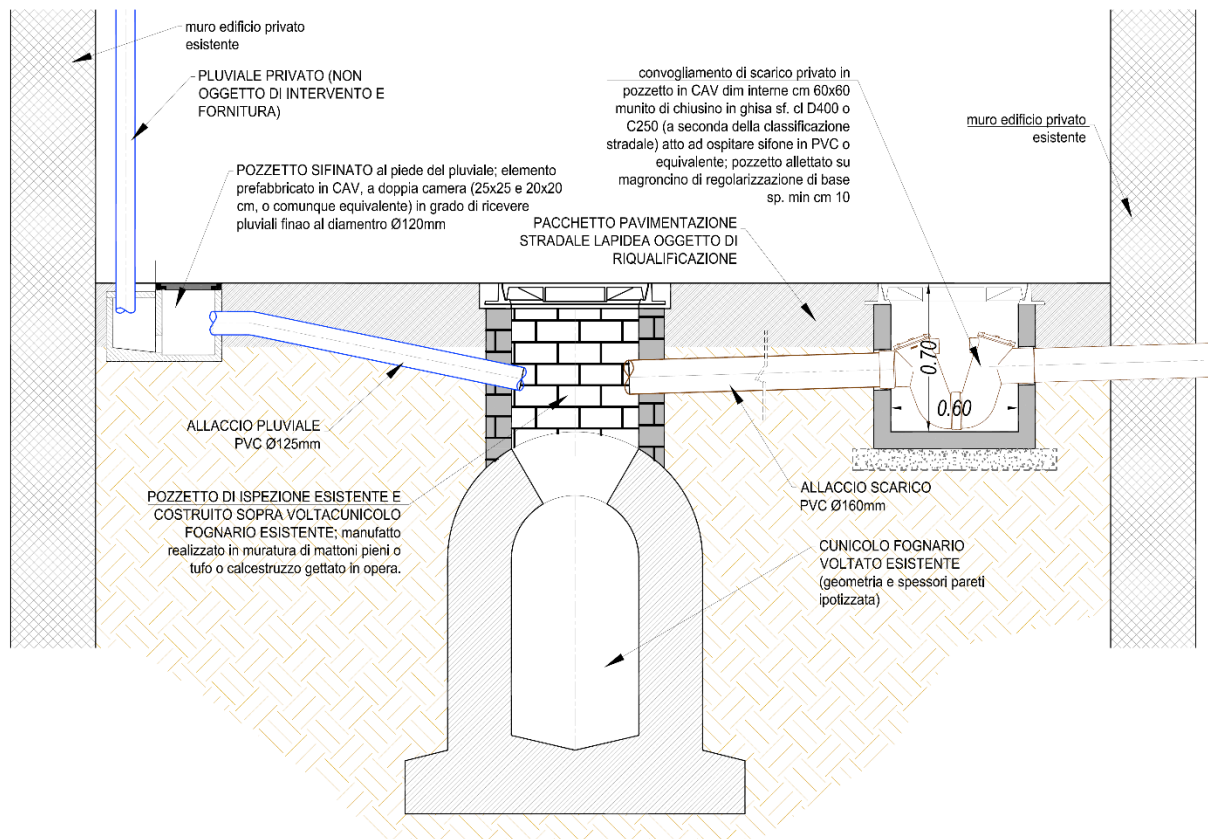
Figura 26 – Cunicolo fognario
