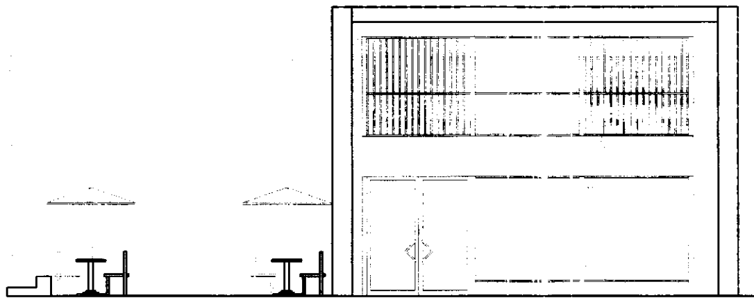
238 PROSPETTO RICADENTE IN GALLERIA PRIVATA (PROIEZIONE DELL'EDIFICIO SOVRASTANTE)
