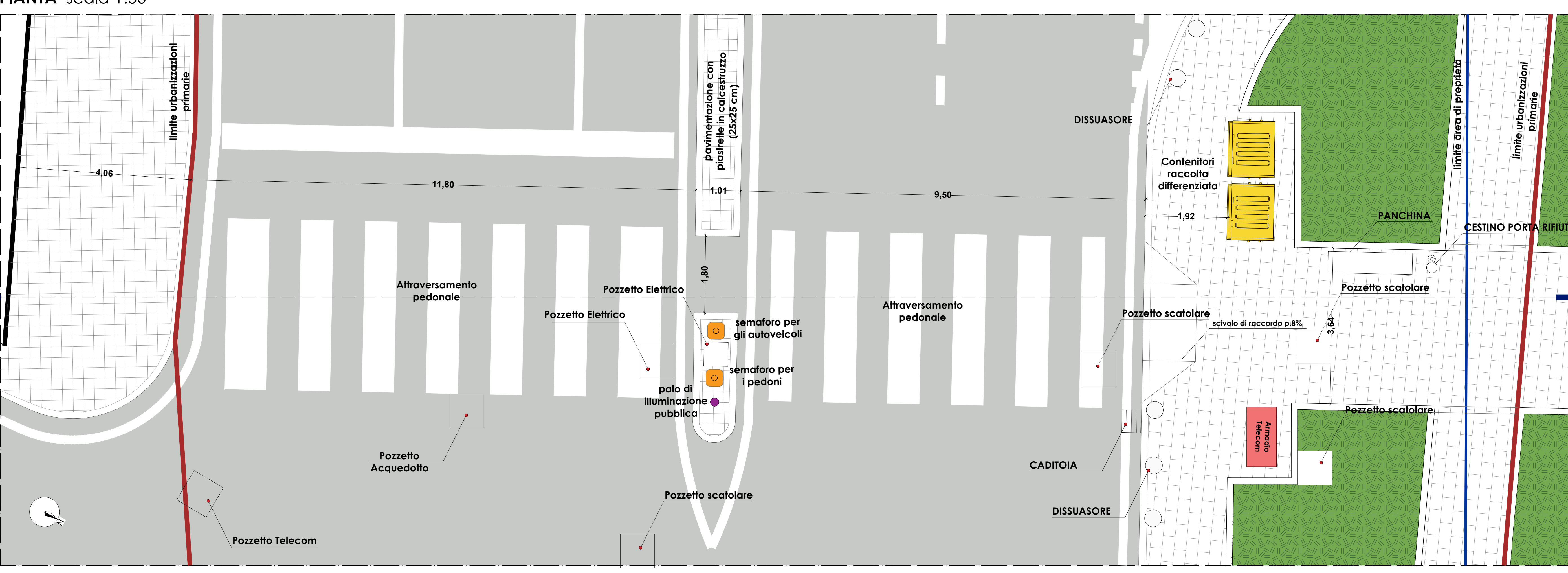
PIANTA scala 1:50
