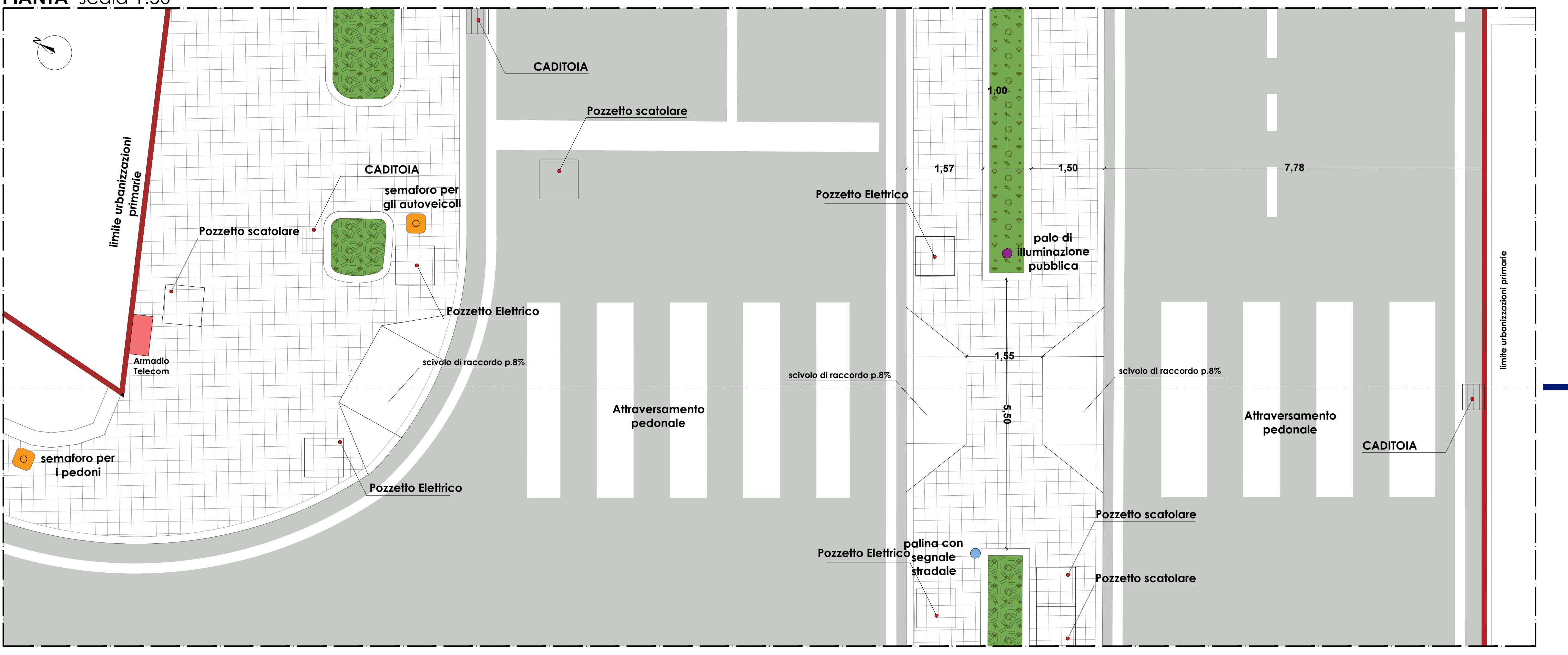
PIANTA scala 1:50
