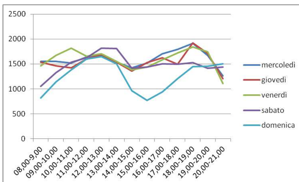
Figura 2.3.1.6 –Auto equivalenti/ora
