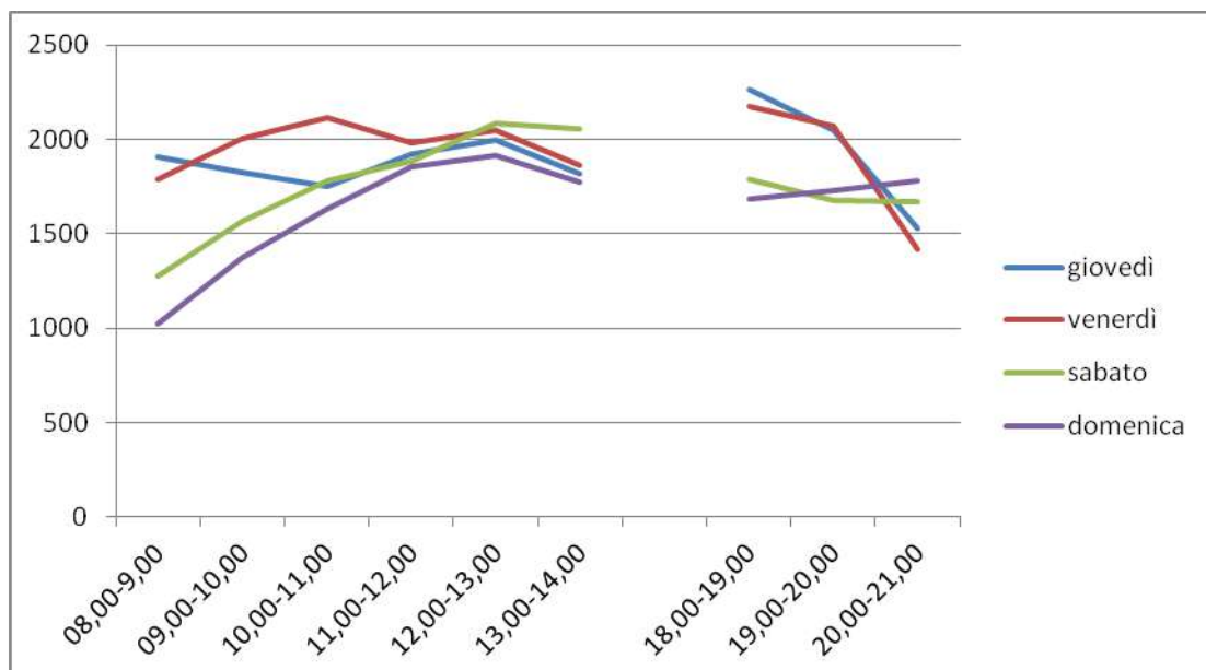
Figura 2.3.8 – Andamento orario dei flussi veicolari equivalenti
