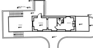
Pianta Piano Terra Rapp. 1:100
