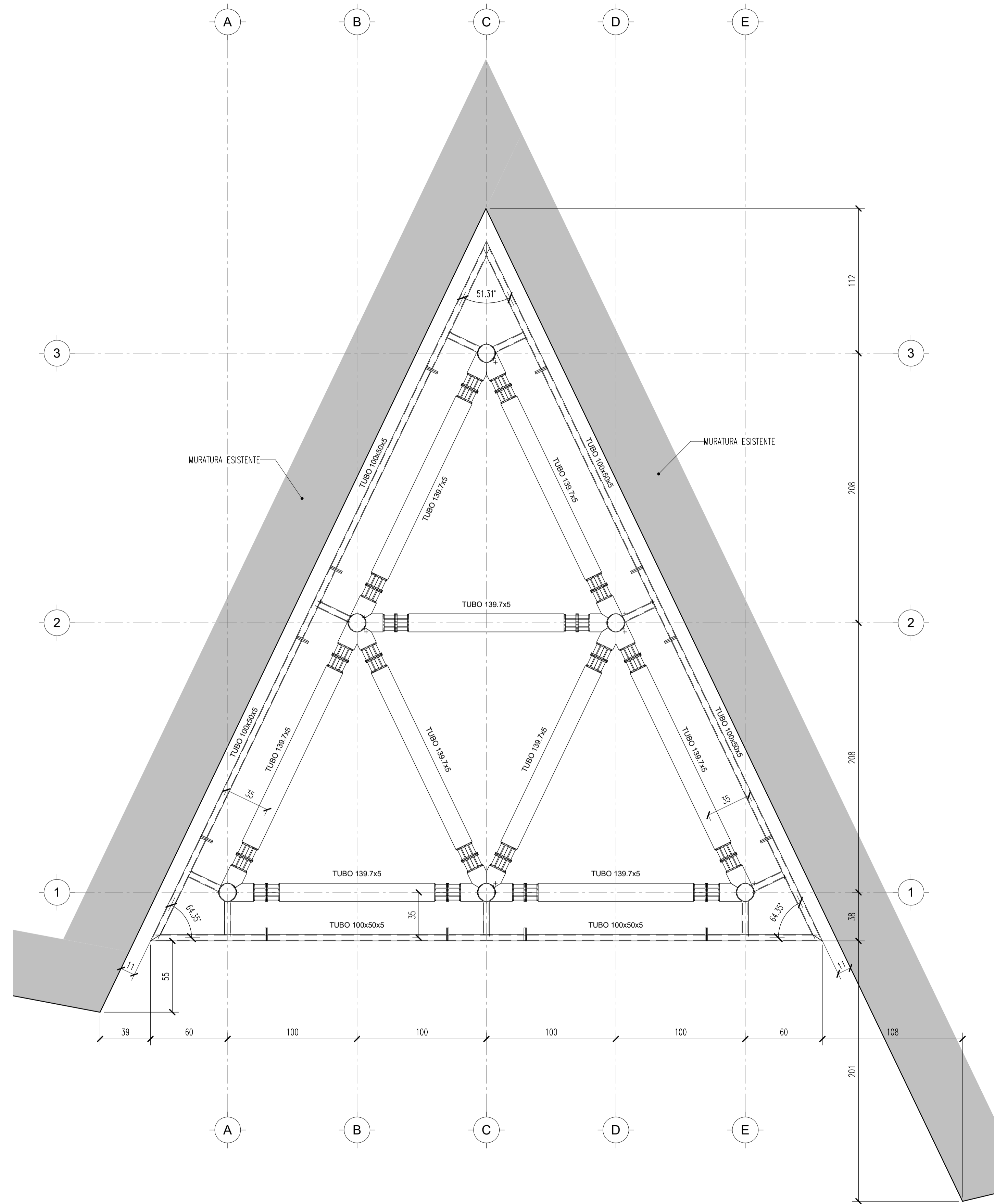
2 Carpenteria - Pianta delle Coperture 1:20
