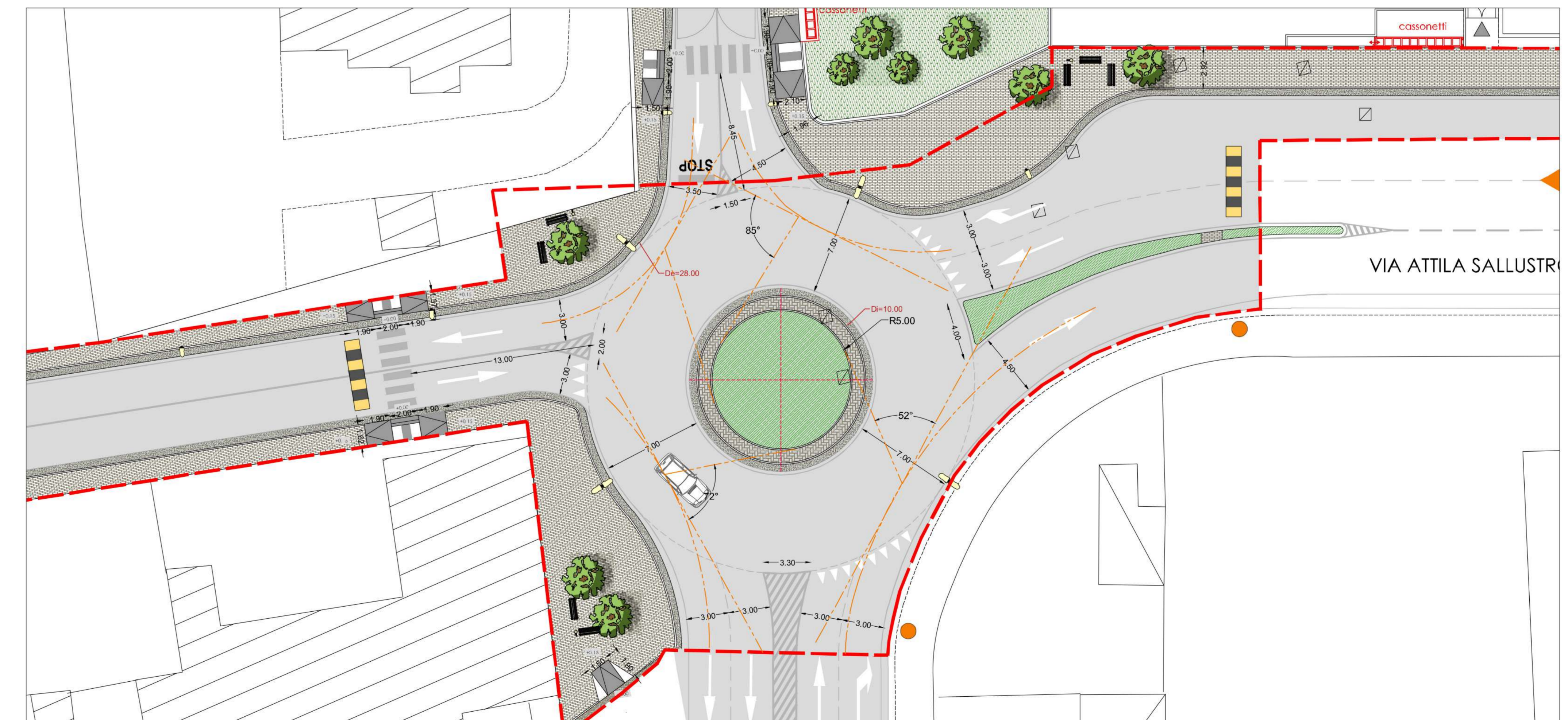
ANGOLI DI DEVIAZIONE
