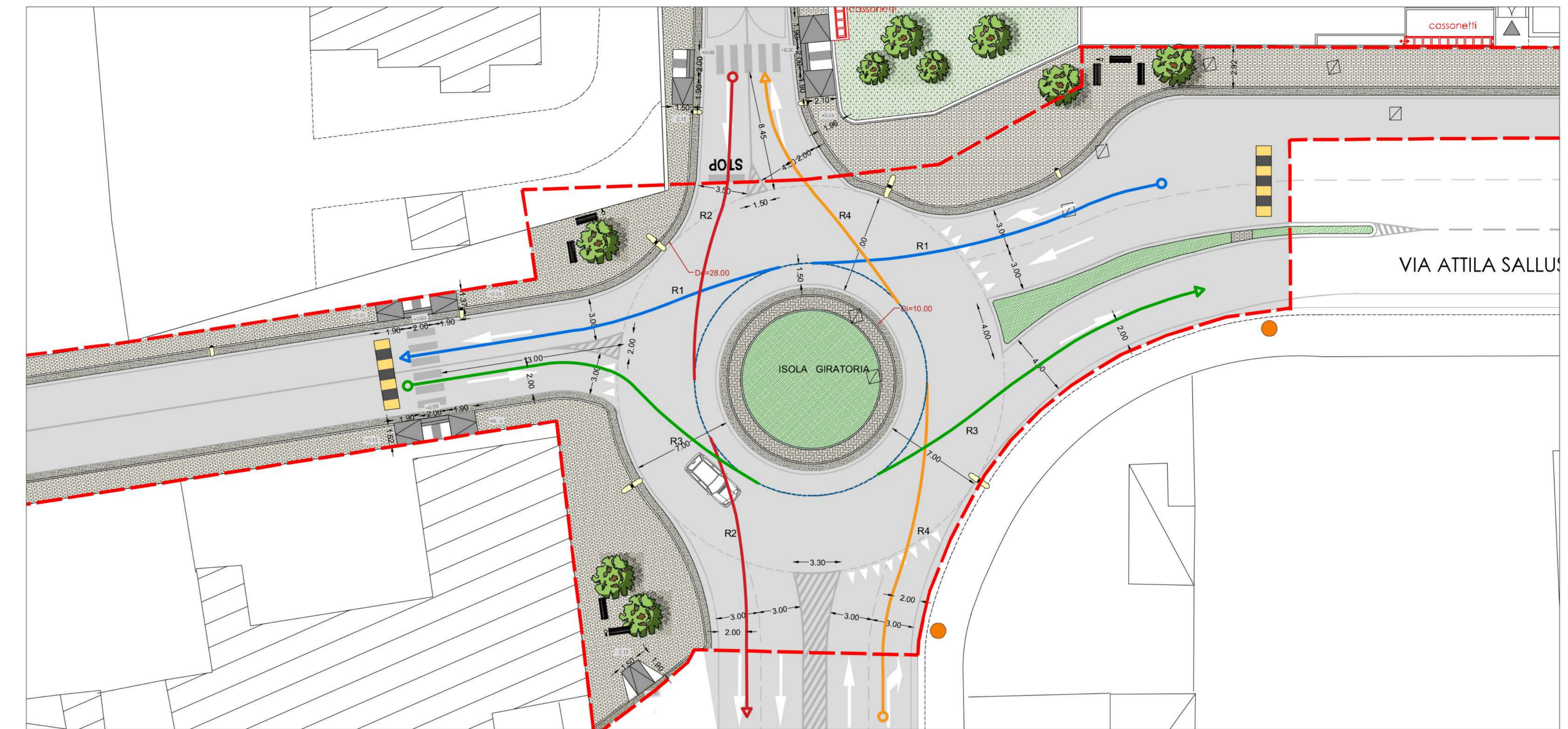
TRAJETTORIE E RAGGI DI DEFLESSIONE
