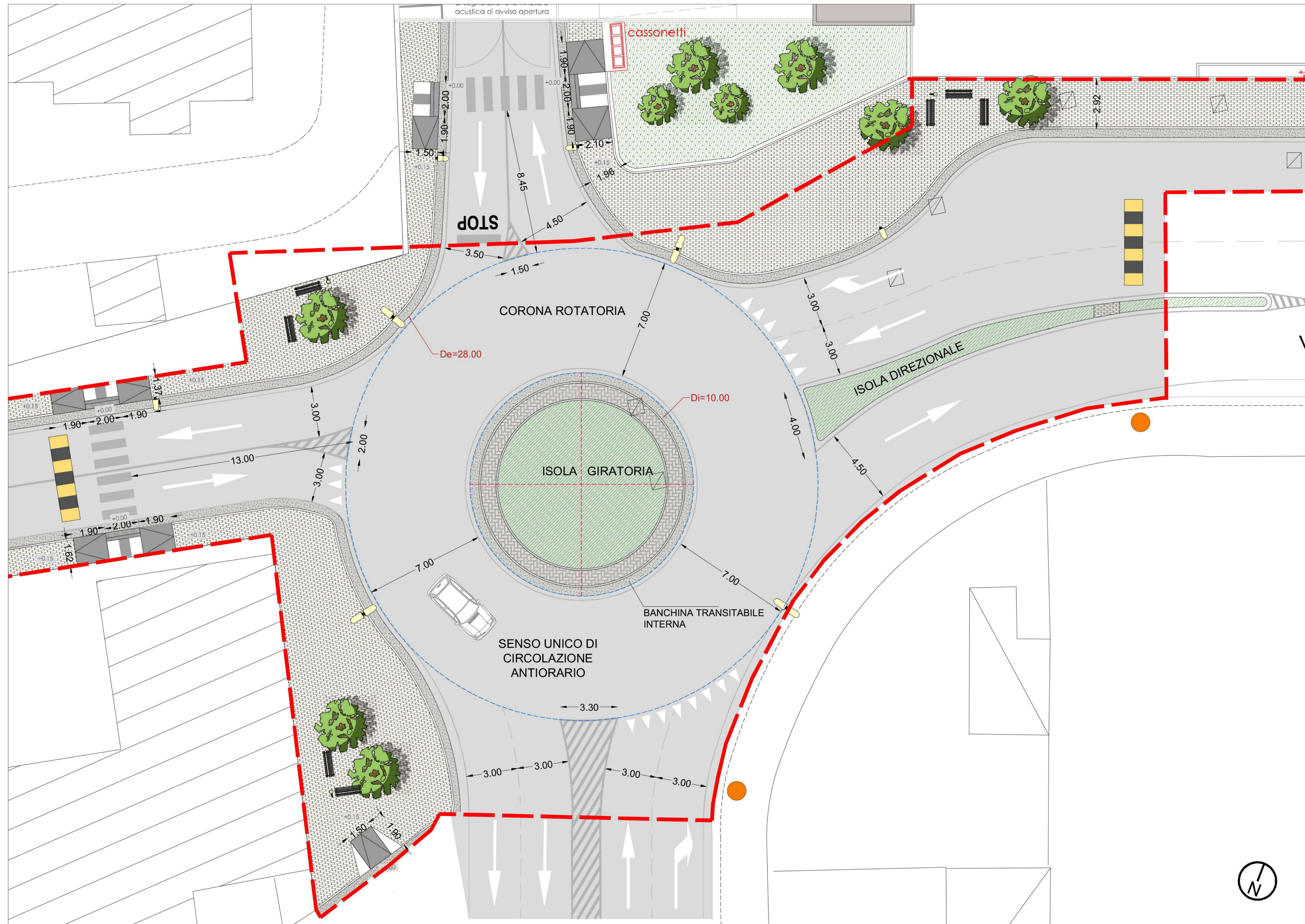
DIMENSIONAMENTO DELLA ROTATORIA
