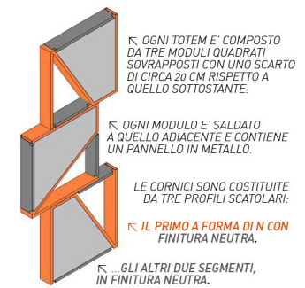
Figura 12_Totem – elaborato esecutivo
