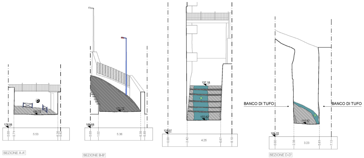
Figura 8 Stralcio elaborato Stato di Conservazione - serie CNAP001GKE – Salita Cacciottoli – Sezioni trasversali
