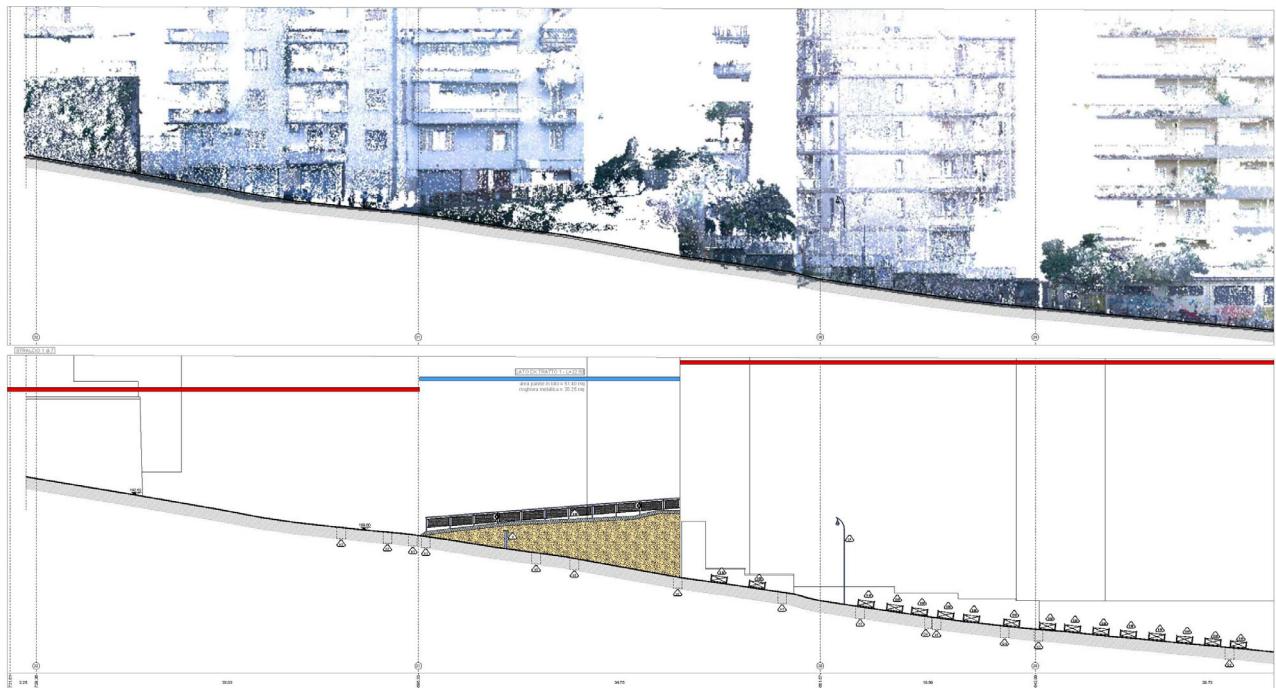
Figura 7 Stralcio elaborato Stato di Conservazione - serie CNAP001GKE- Salita Cacciottoli – Sezione longitudinale
