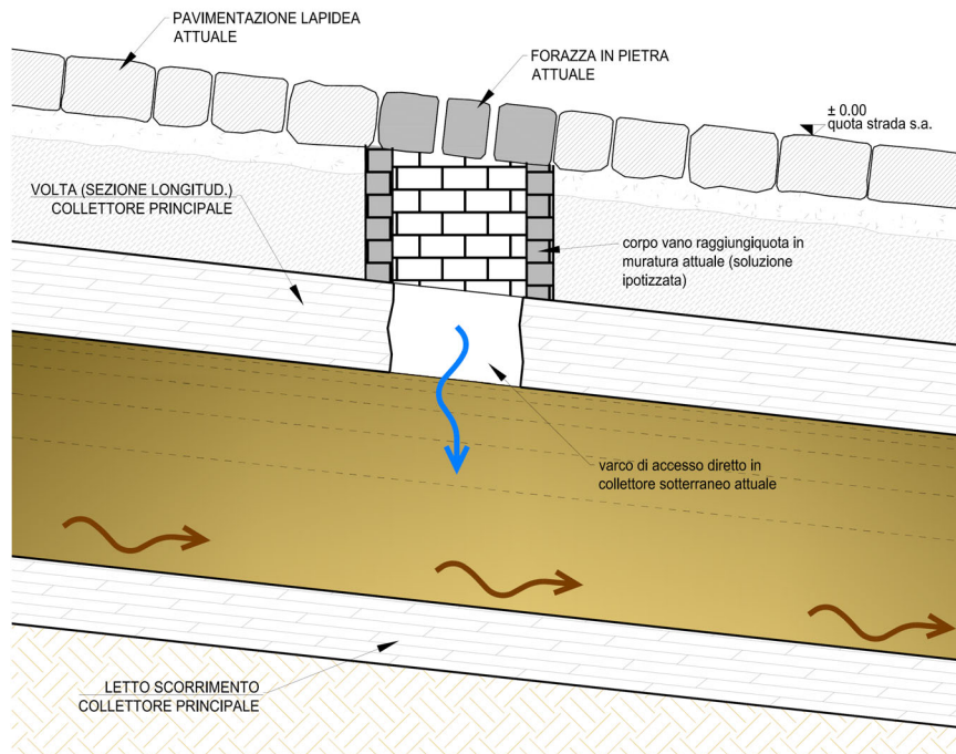
Figura 21 - stato attuale caditoia storica a fessura
