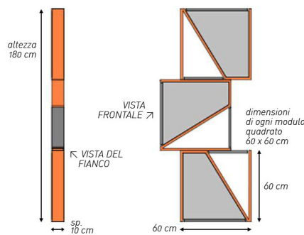
Figura 12_Totem – elaborato esecutivo
