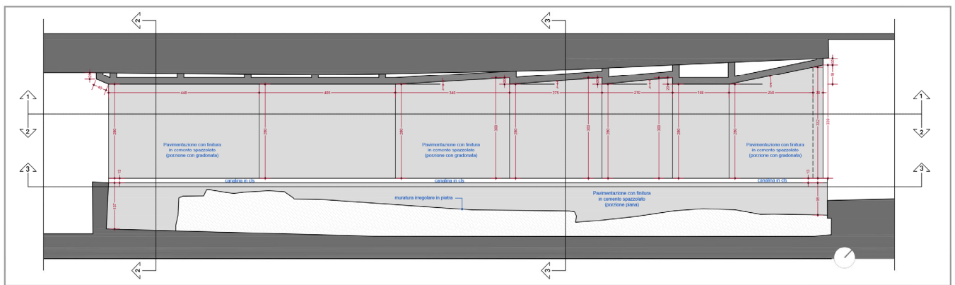
Figura 13 Pianta
