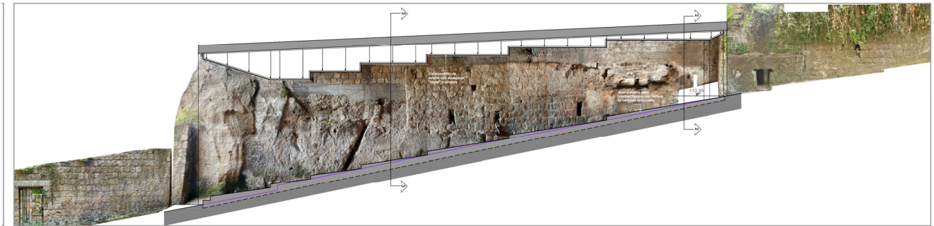
Figura 15 Sezione longitudinale 2-2
