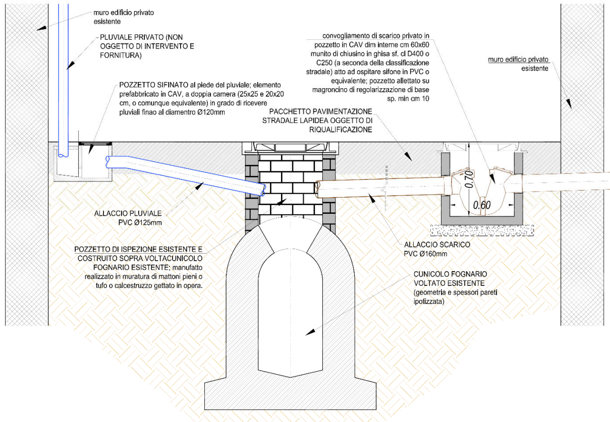
Figura 25 - Cunicolo fognario
