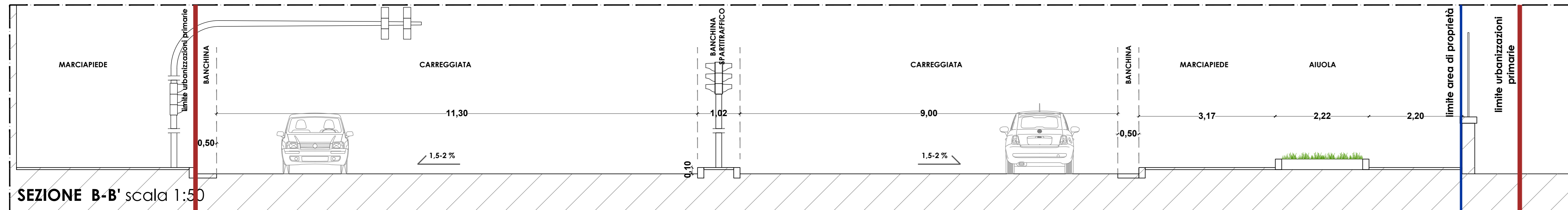
SEZIONE B-B' scala 1:50
