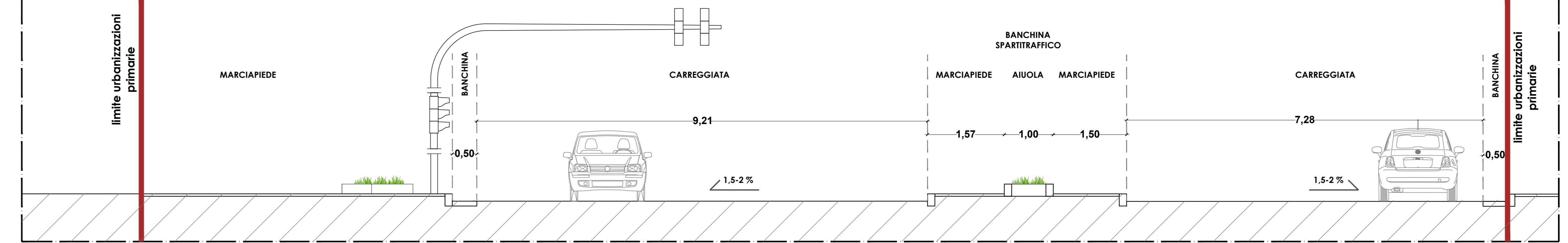
SEZIONE C-C' scala 1:50
