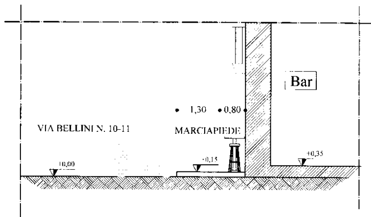
Sezione A:A' "Stato di Progetto" scala 1:100
