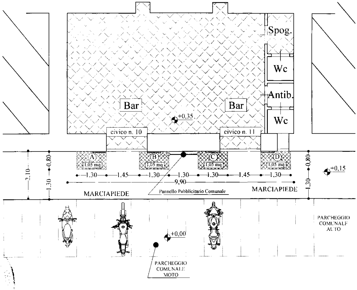
Planimetria "Stato di Progetto" scala 1:100
