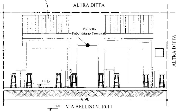
Prospetto "Stato di Progetto" scala 1:100
