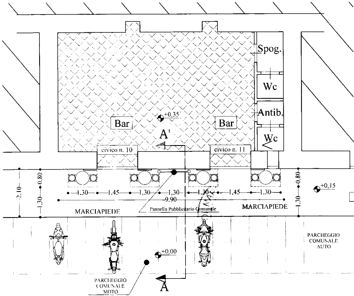
Planimetria "Stato di Progetto" scala 1:100
