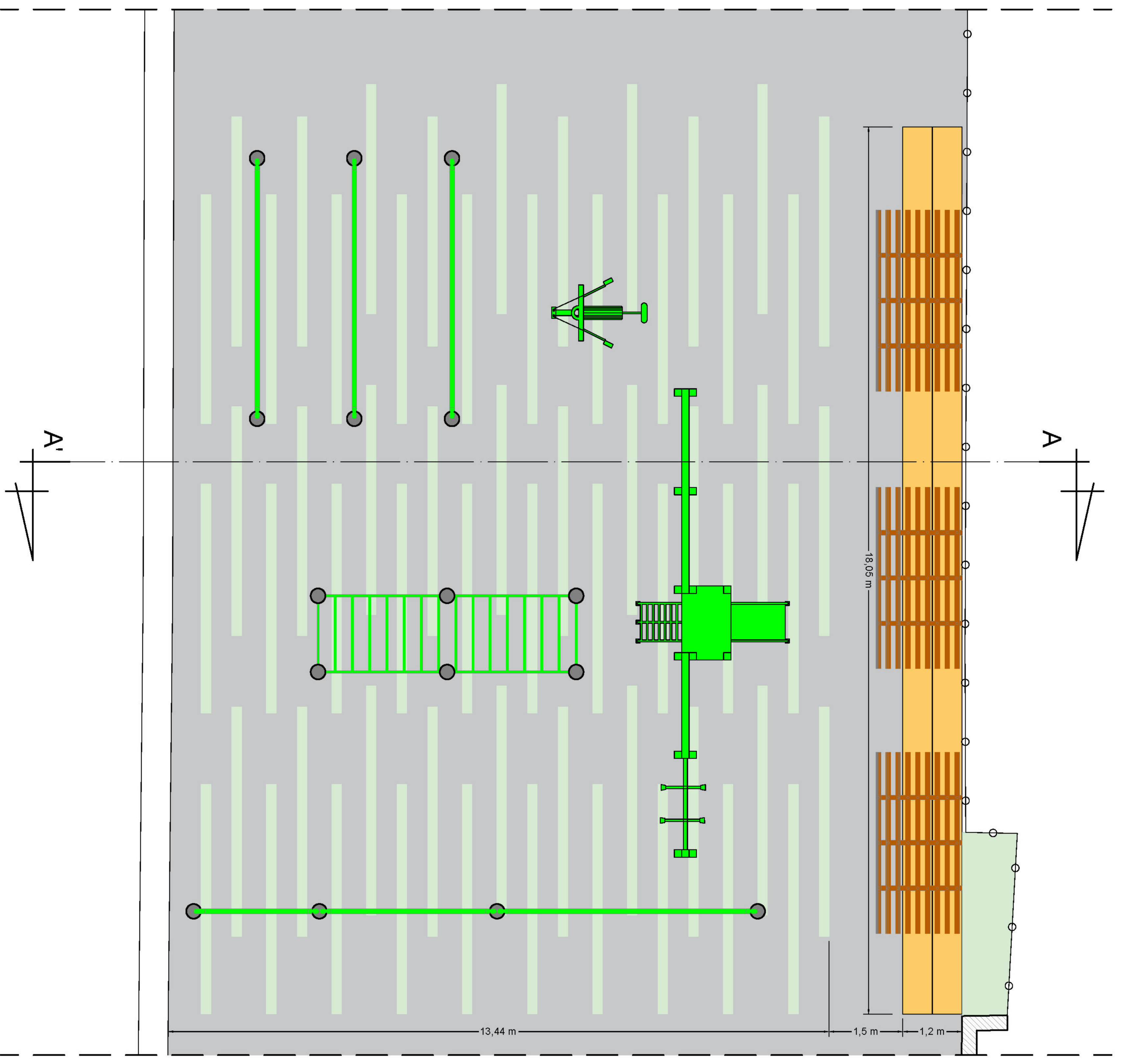
Pianta di dettaglio percorso fitness (area 4) - Scala 1:50
