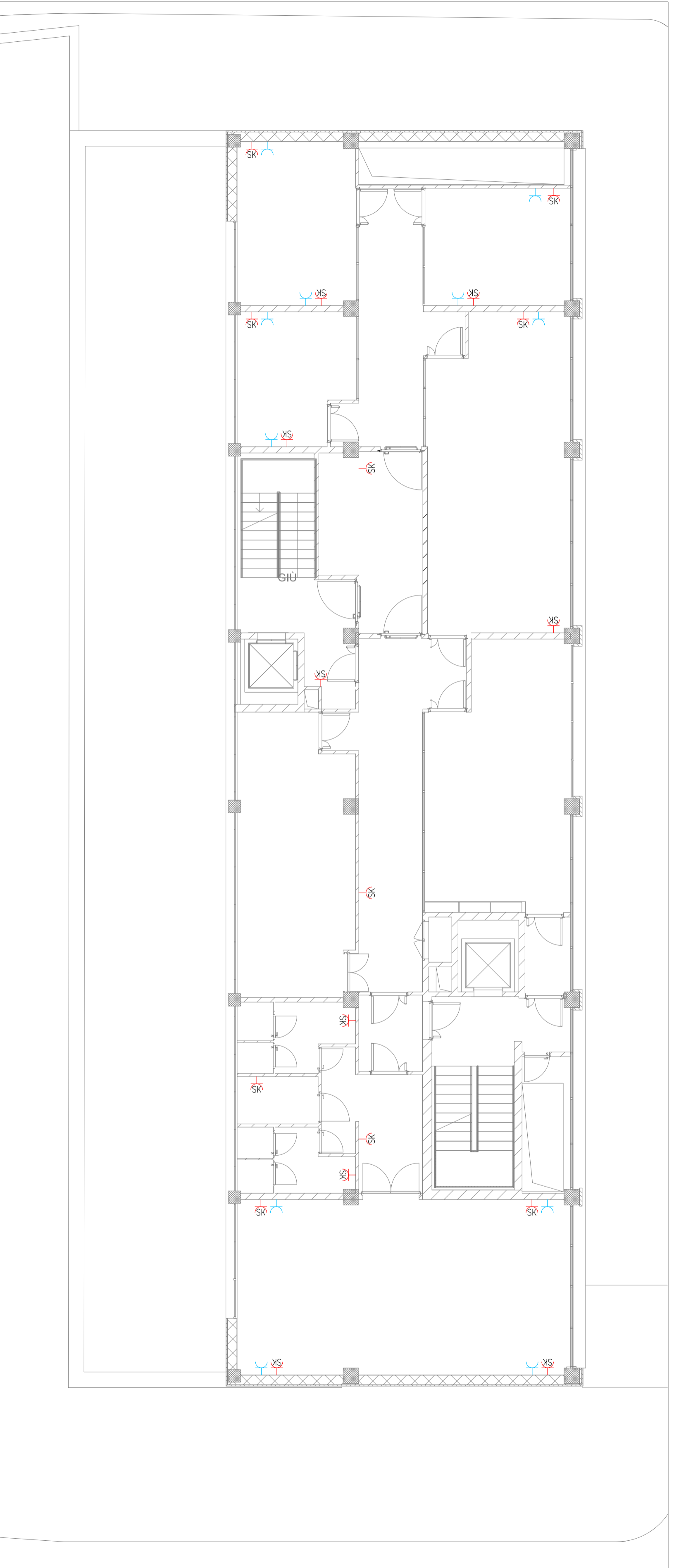
LIVELLO 7.50 - SCALA 1:100
