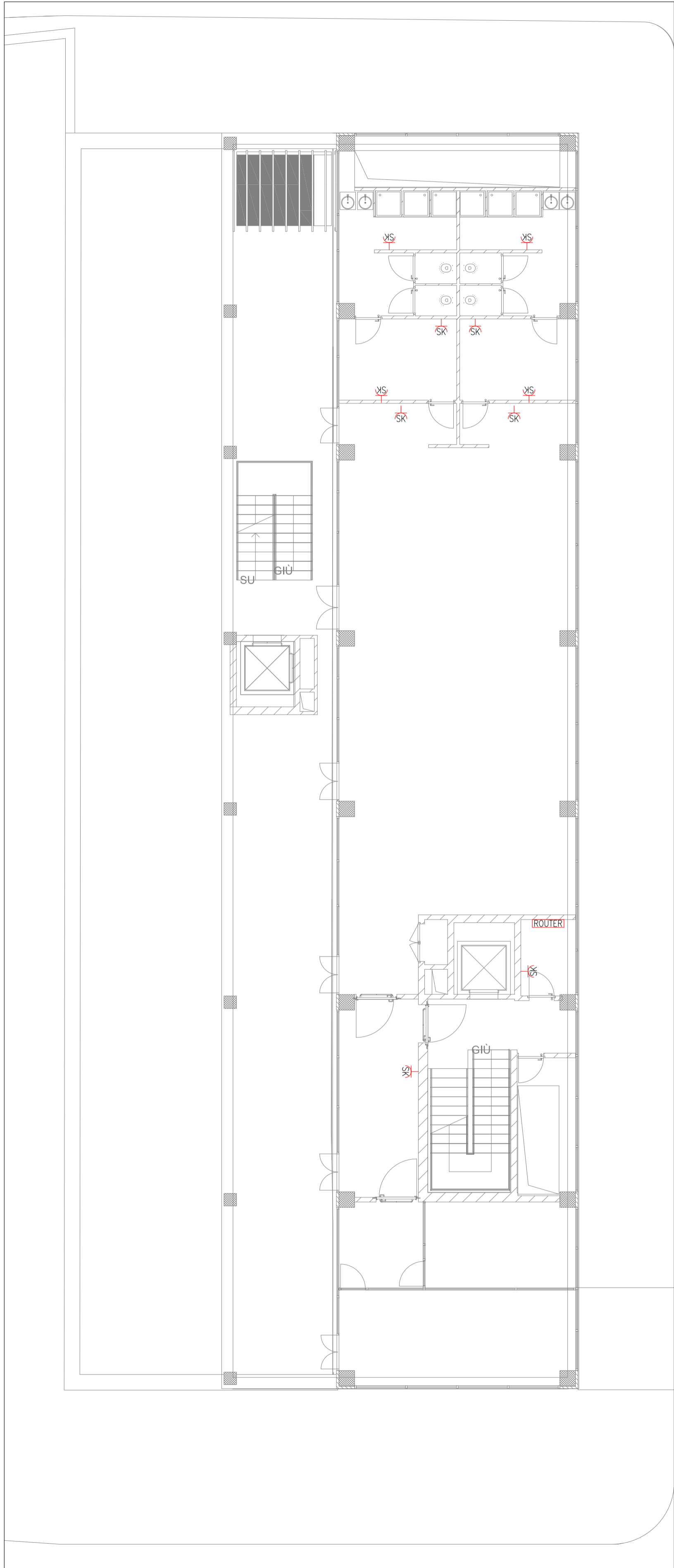
LIVELLO 4.10 - SCALA 1:100
