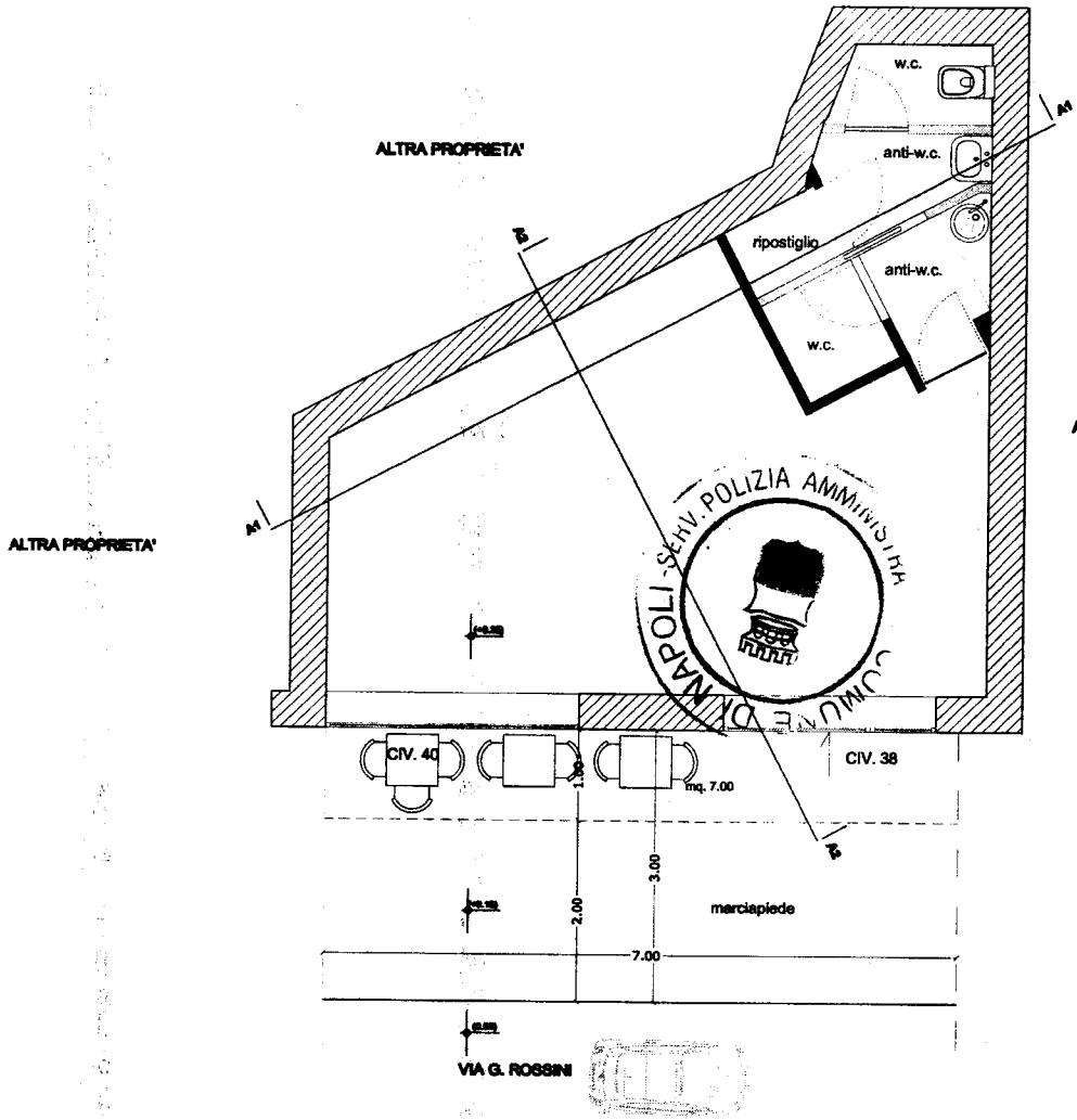
PLANIMETRIA
