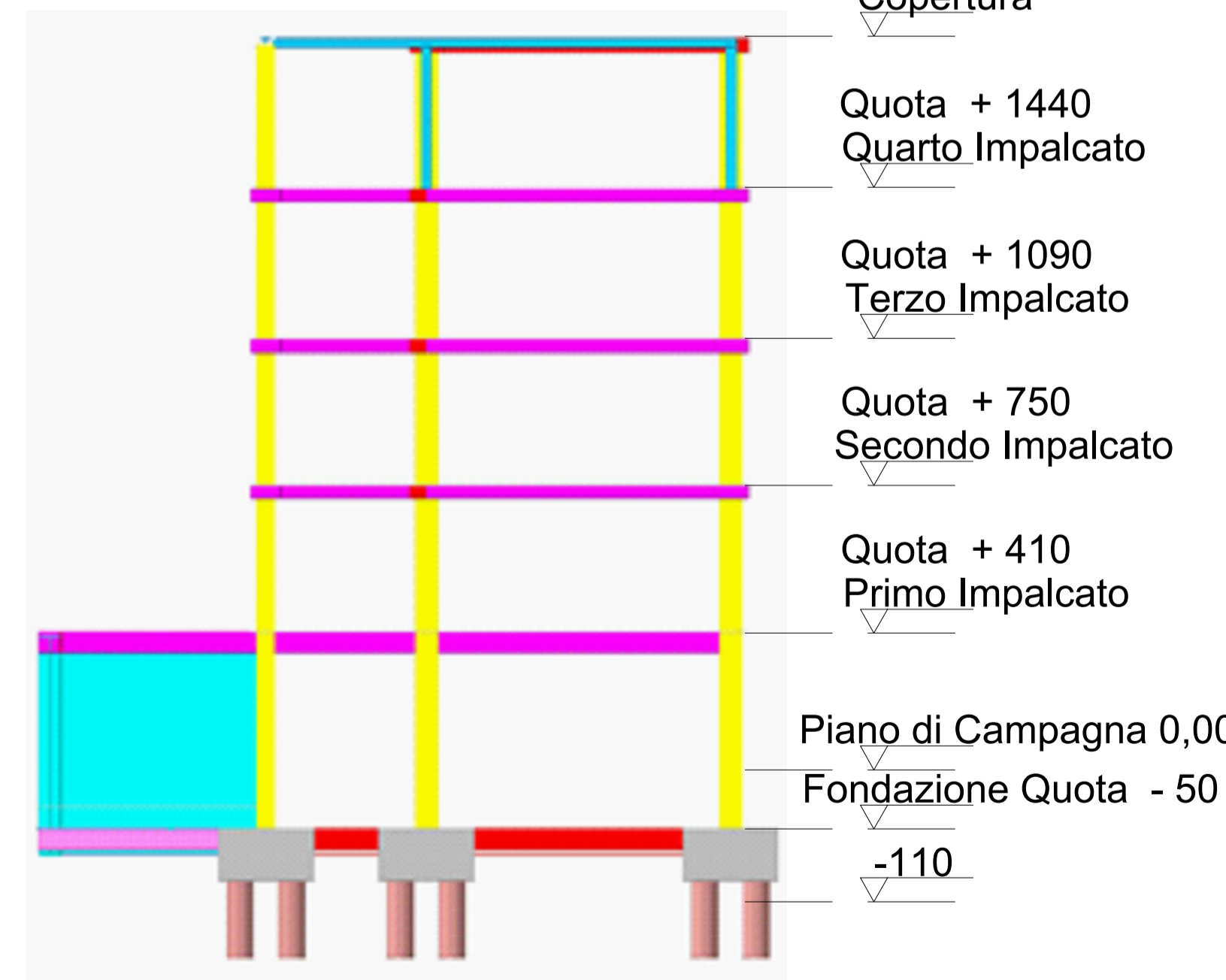
SEZIONE STRUTTURALE
