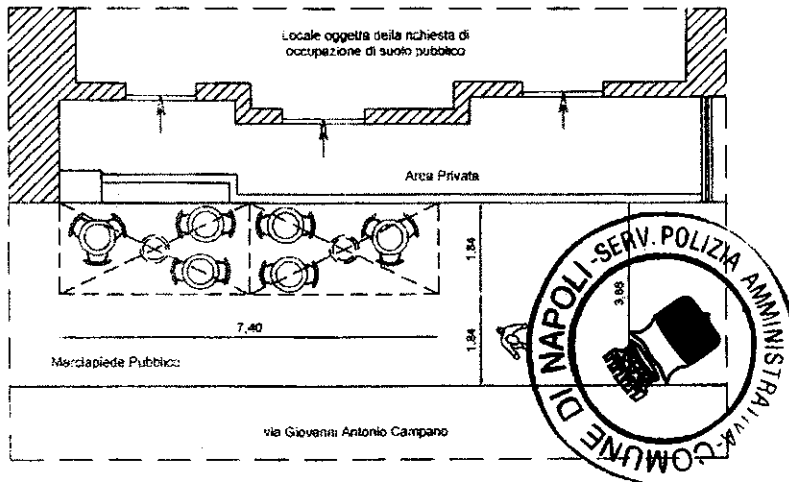
PIANTA Stato di progetto scala 1:100
