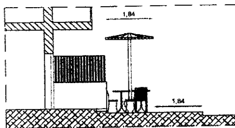
SEZIONE Stato di Progetto Scala 1:100
