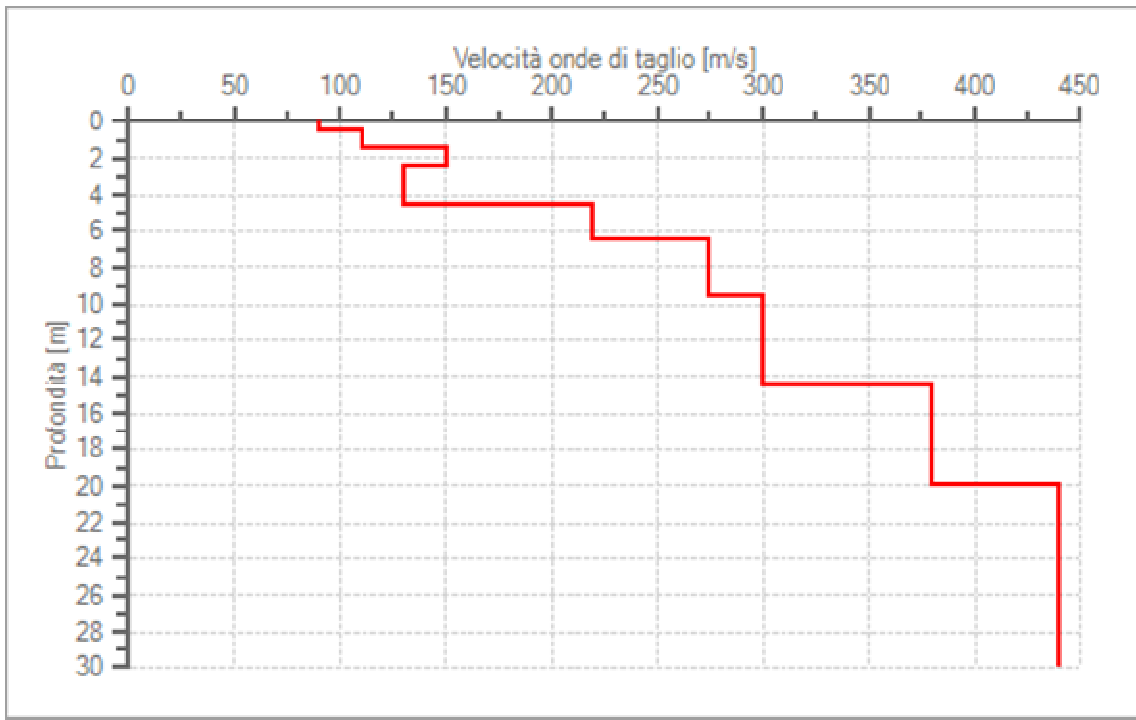
Fig. 14 - Profilo delle velocità delle onde di taglio.
