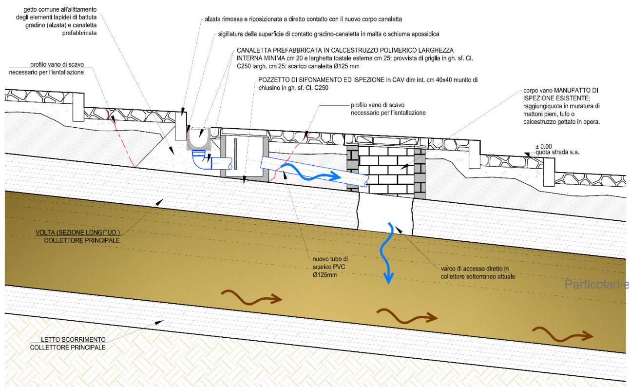
Figura 21 - inserimento di canalette a ridosso delle alzate gradinate esistenti
