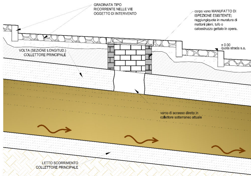
Figura 19 - torrino di ispezione tipo
