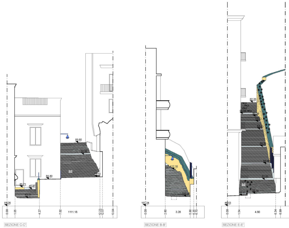
Figura 8 Stralcio elaborato Stato di Conservazione - serie CNAP001GKE – Calata San Francesco – Sezioni
