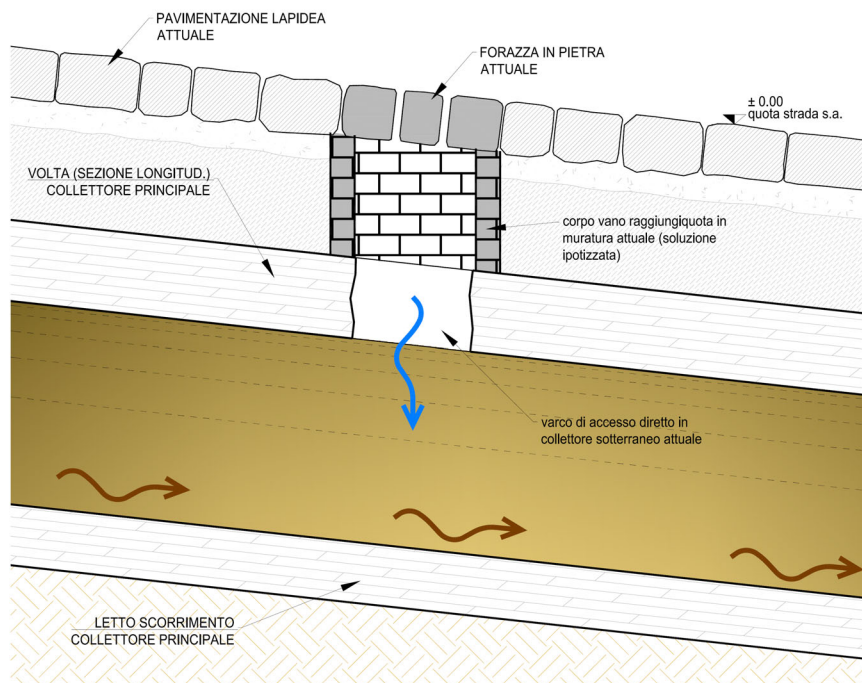
Figura 18 - stato attuale caditoia storica a fessura
