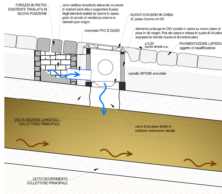
Figura 20 - soluzione spostamento caditoia storica a fessura e suo sifonamento
