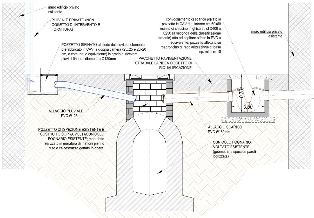
Figura 22 - Cunicolo fognario
