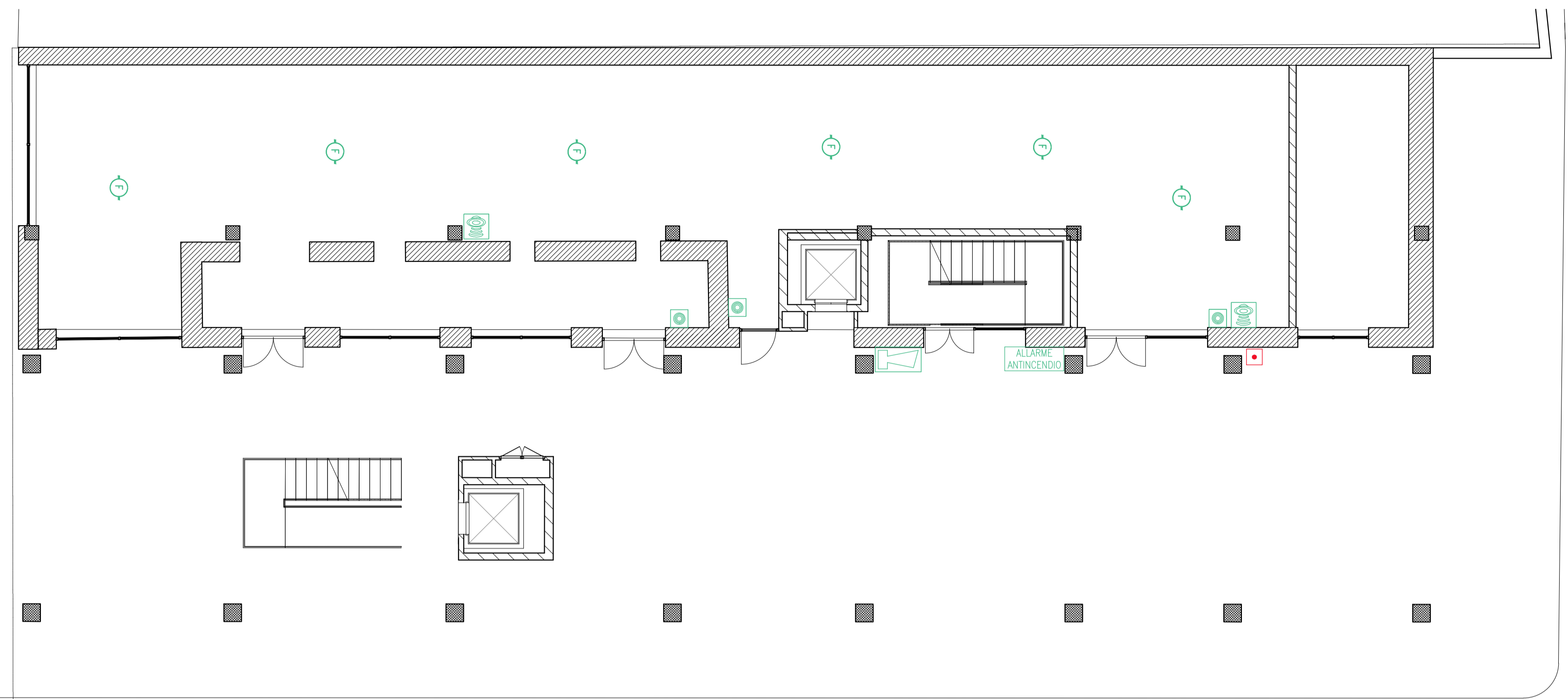
PIANTA PIANO TERRA - CORPO ALTO - NEGOZI DI VICINATO sc.1:100
