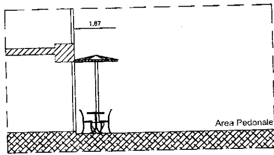
SEZIONE Stato di progetto Scala 1:100
