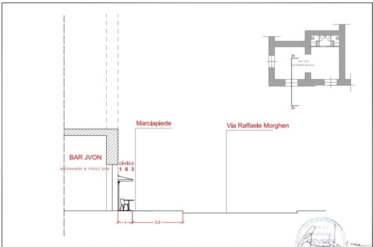
Sezione AA - Progetto
