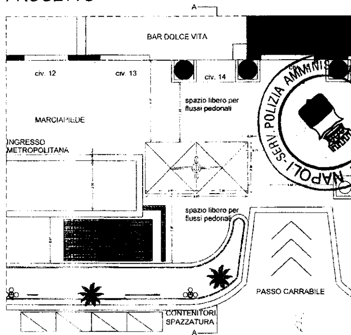
PLANIMETRIA PIANO TERRA SCALA 1:100
