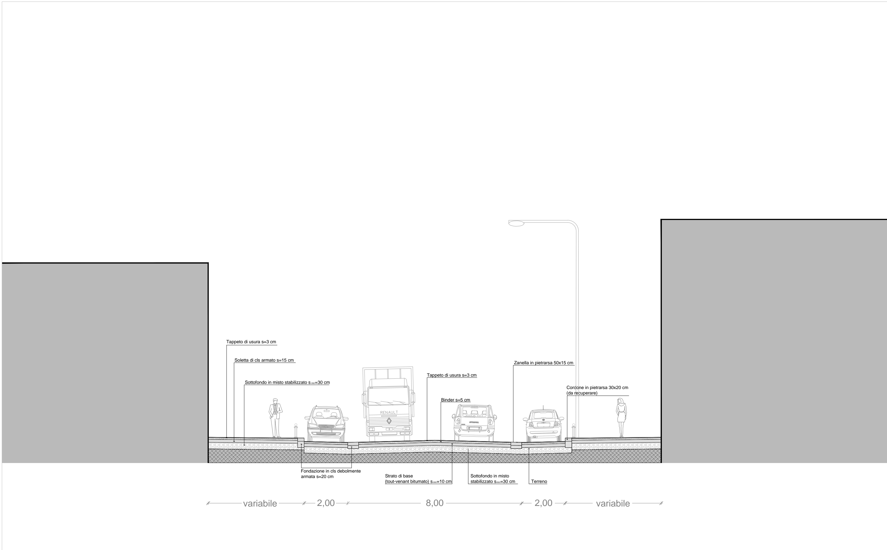
Via Brecece a Sant'Erasmo - sezione tipo, scala 1:100
