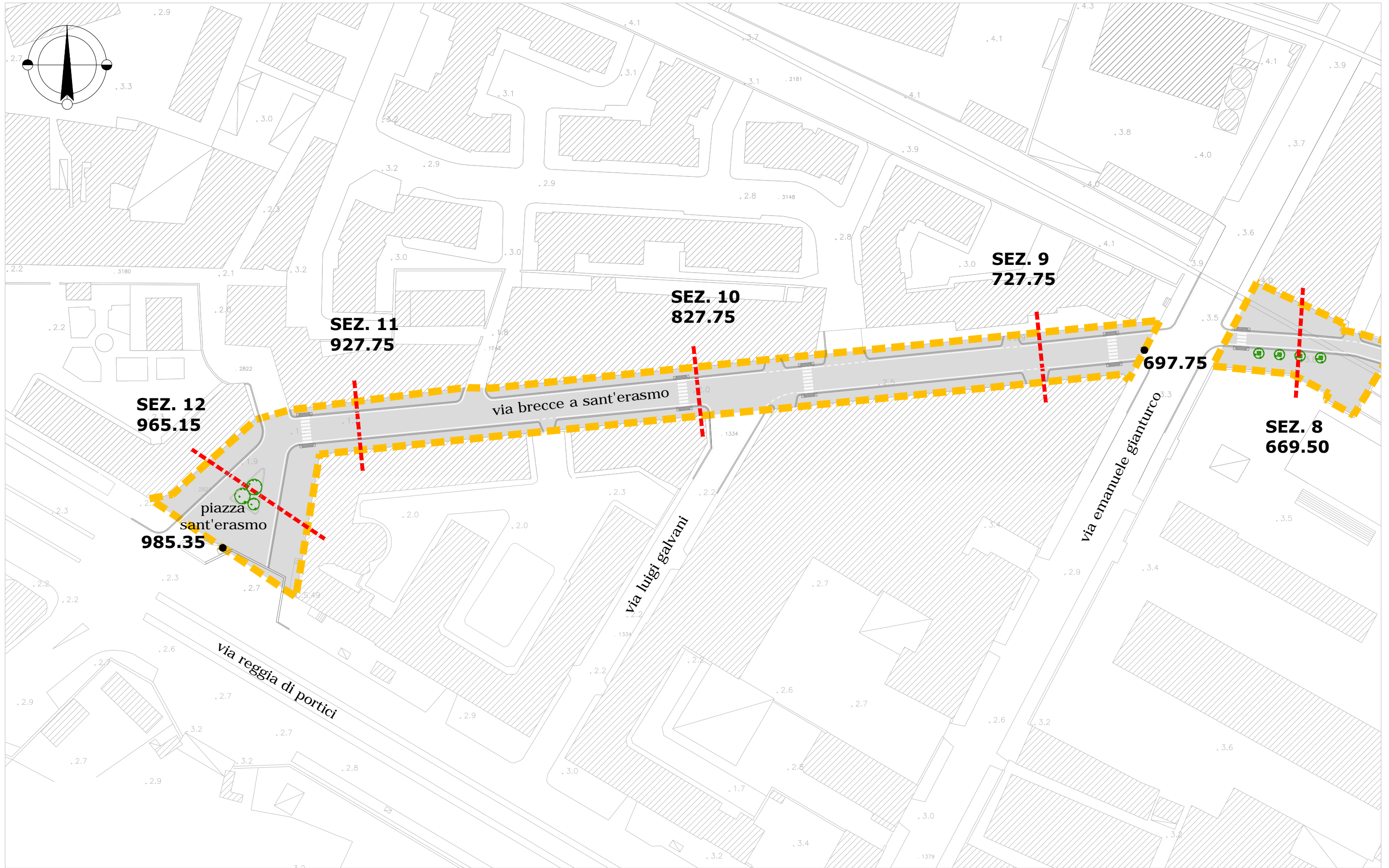
Via Brece a Sant'Erasmus, tratta via Emanuele Gianturco/piazza Sant'Erasmus - planimetria scala 1:1000
