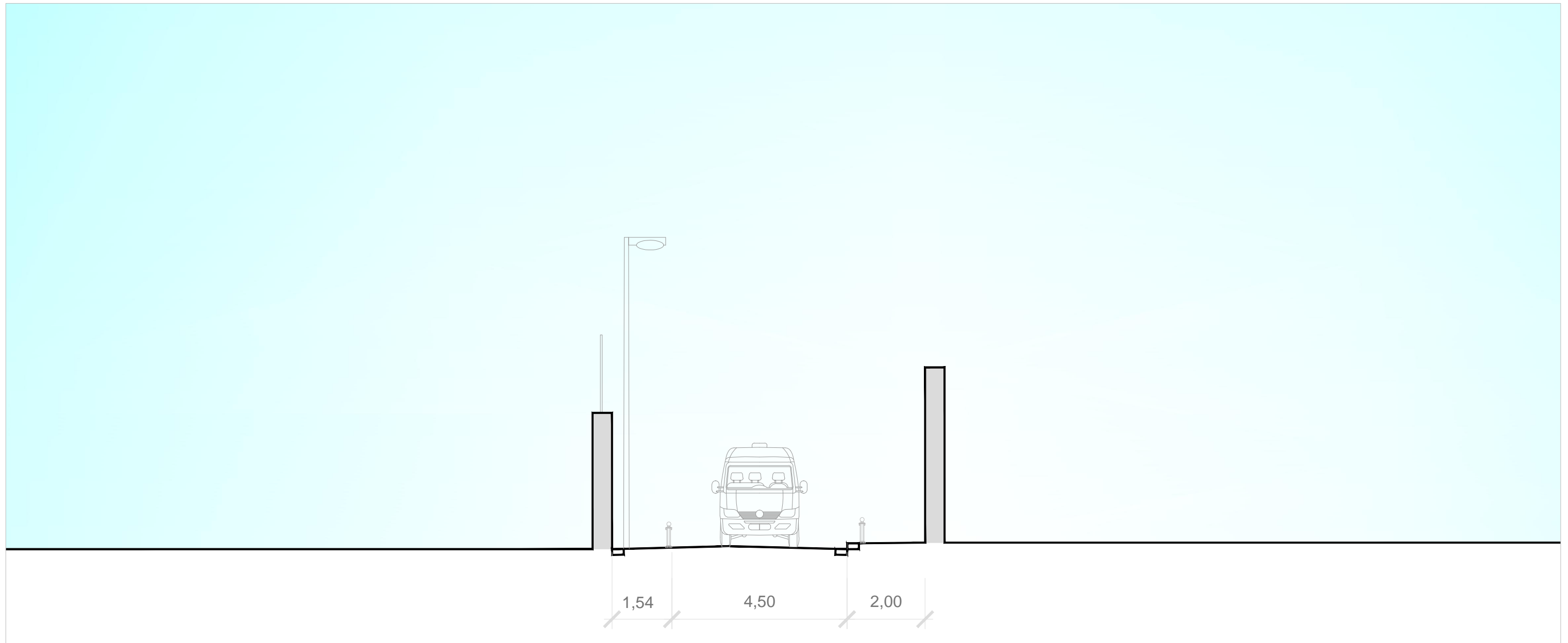
Via Brece a Sant'Erasmus, tratta via Irpinia/via Emanuele Gianturco - SEZ. 7, scala 1:100
