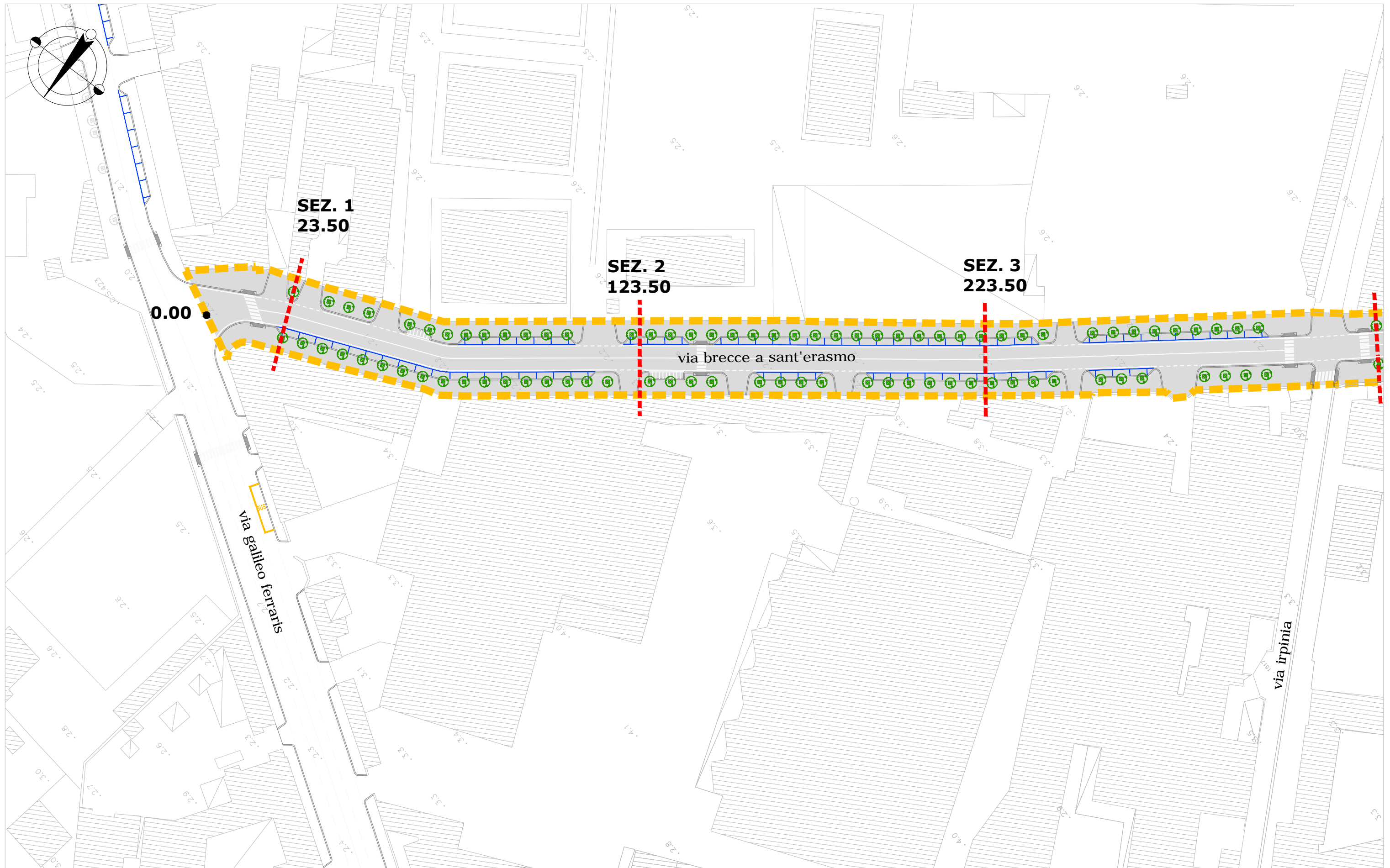
Via Brece a Sant'Erasmus, tratta via Galileo Ferraris/via Irpinia - planimetria scala 1:1000
