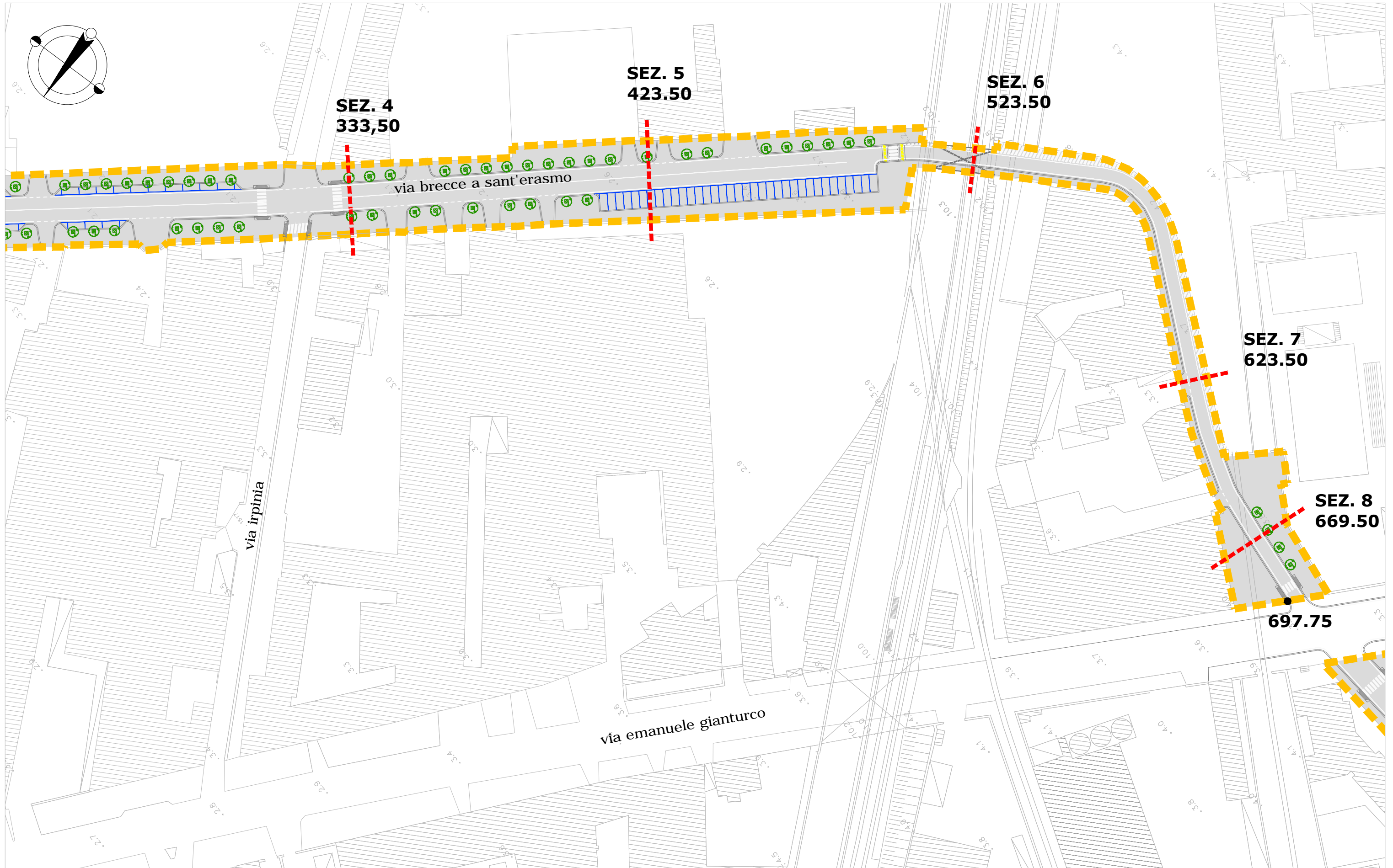
Via Brece a Sant'Erasmus, tratta via Irpinia/via Emanuele Gianturco e via Irpinia - planimetria scala 1:1000
