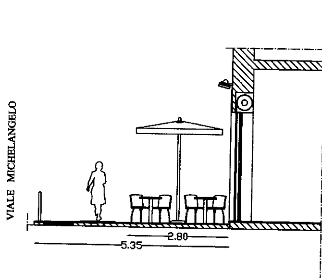
SEZIONE DI PROGETTO DELL'AREA INTERESSATA SCALA 1:100
