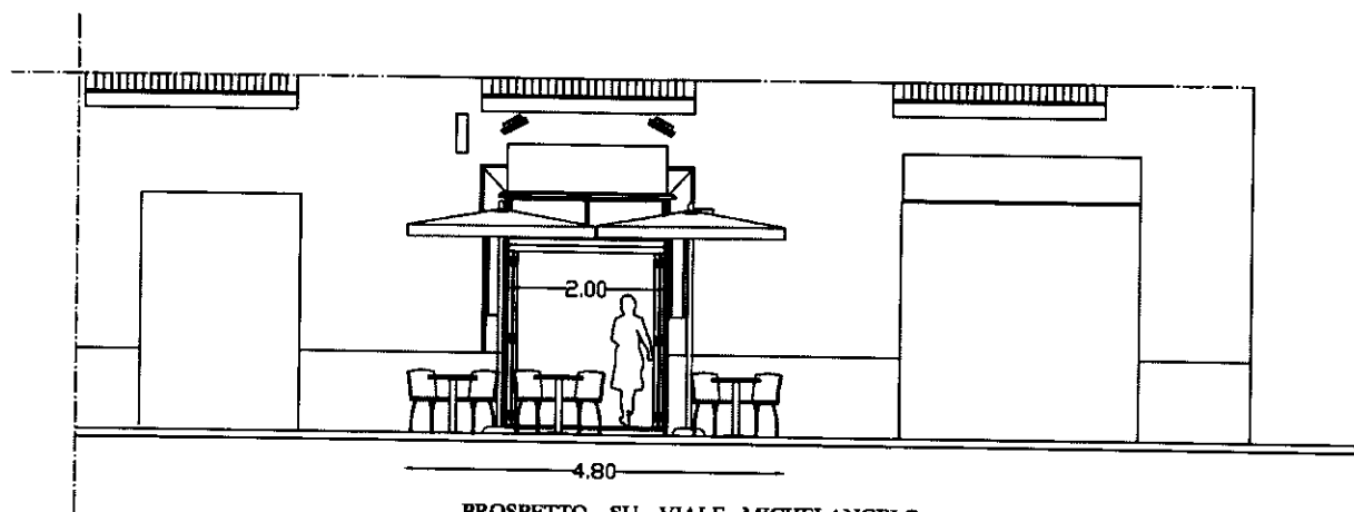
PROSPETTO SU VIALE MICHELANGELO PROSPETTO DI PROGETTO DELL'AREA INTERESSATA SCALA 1:100
