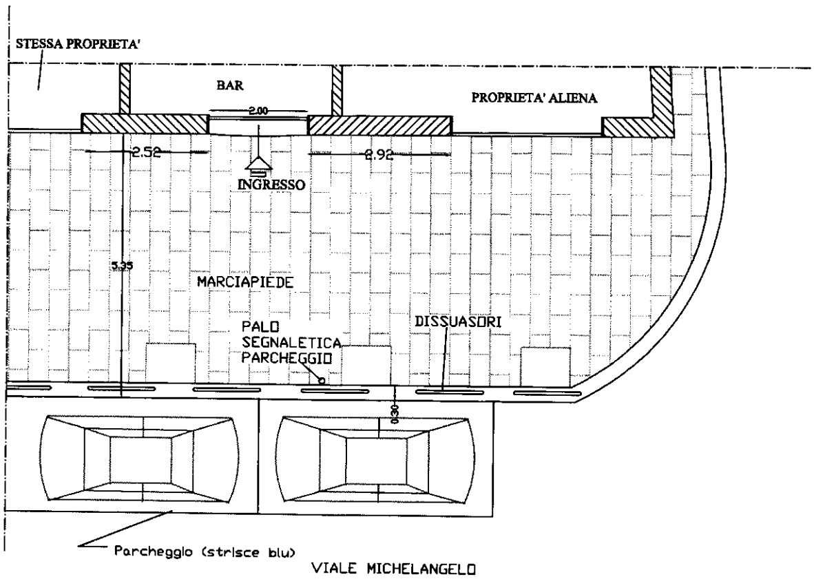
PLANIMETRIA DI RILIEVO DELL'AREA DA OCCUPARE SCALA 1:100
