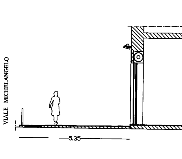
SEZIONE DI RILIEVO DELL'AREA INTERESSATA SCALA 1:100
