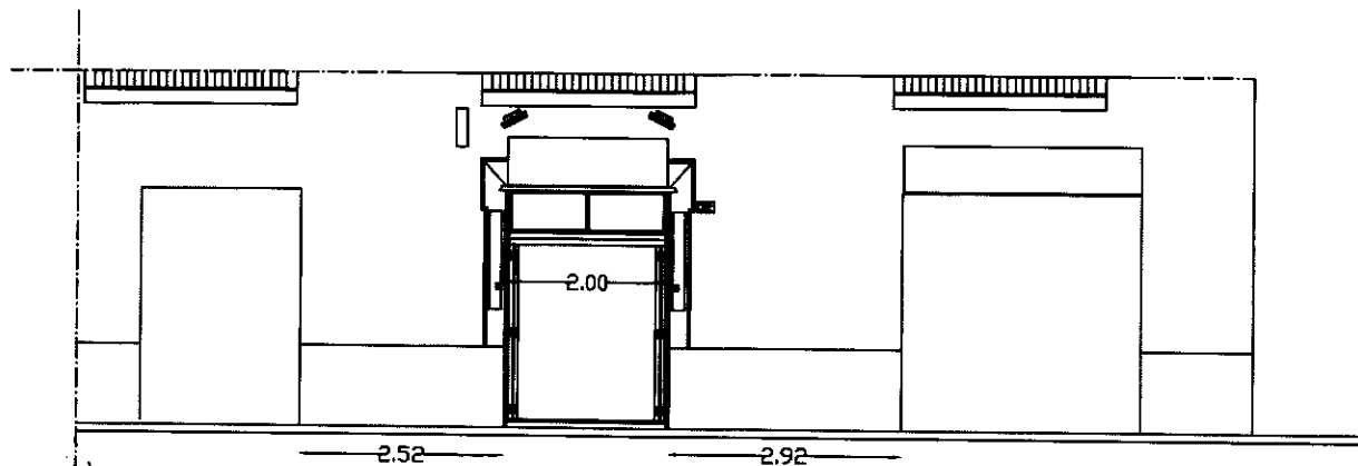
PROSPETTO SU VIALE MICHELANGELO PROSPETTO DI RILIEVO DELL'AREA INTERESSATA SCALA 1:100
