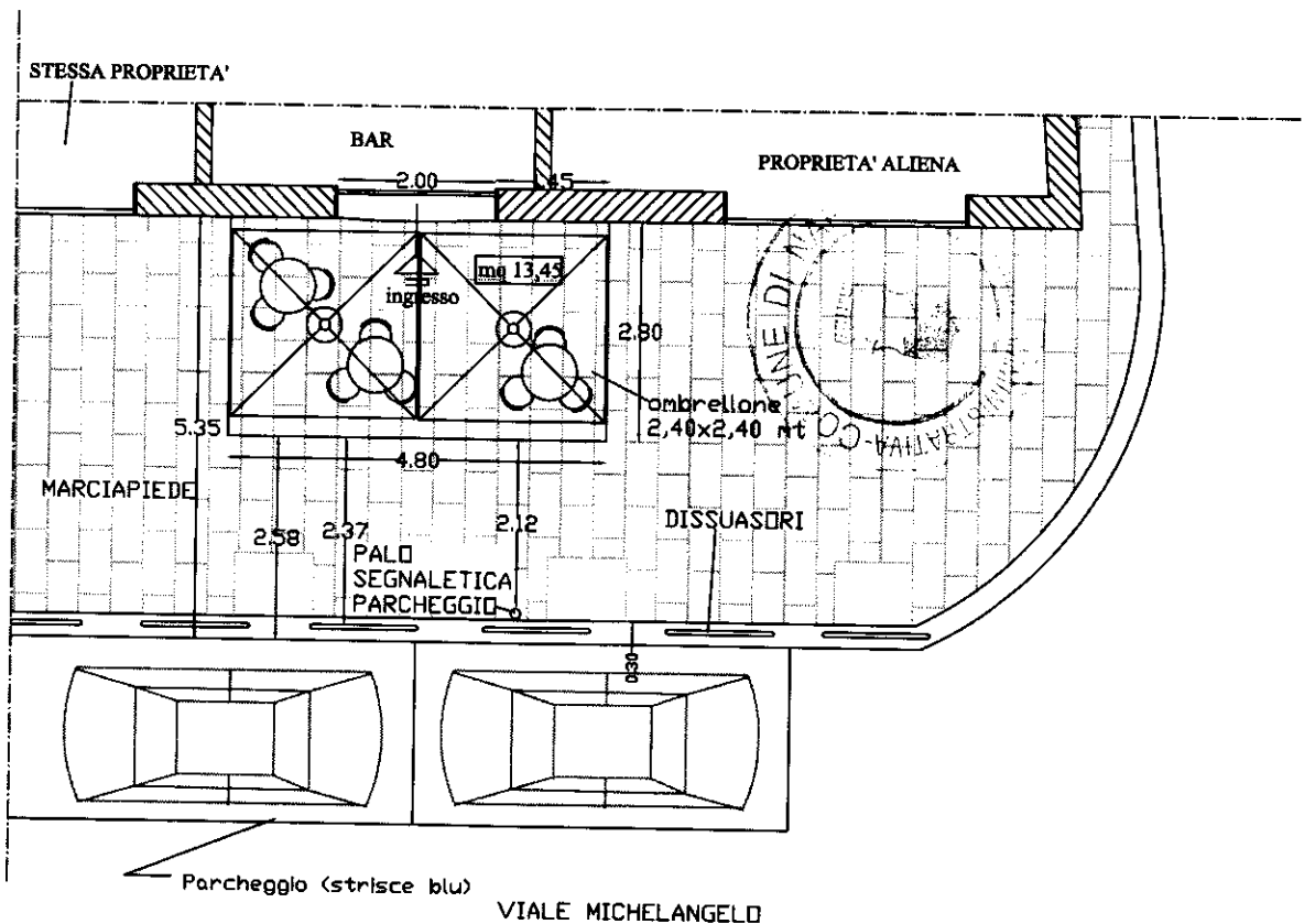
PLANIMETRIA DI PROGETTO DELL'AREA DA OCCUPARE SCALA 1:100
