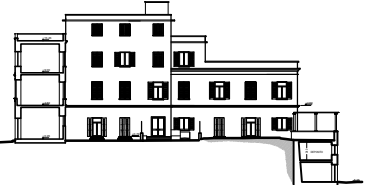
PROSPETTO - SEZIONE 5 Scale 1:200
