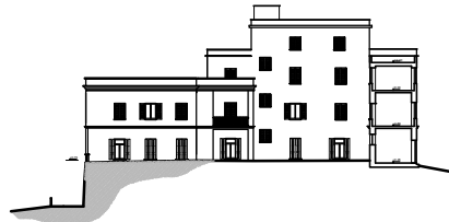
PROSPETTO - SEZIONE 6 Scale 1:200
