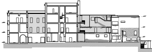
PROSPETTO - SEZIONE 7 Scale 1:200
