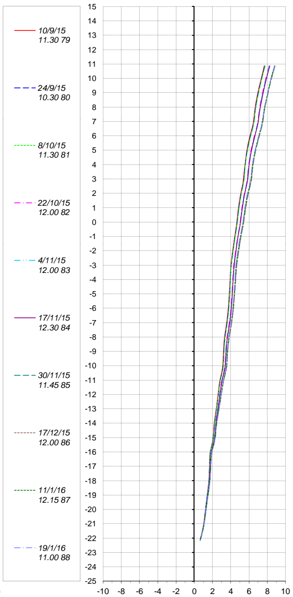
Accorciamento/Allungamento [mm]
