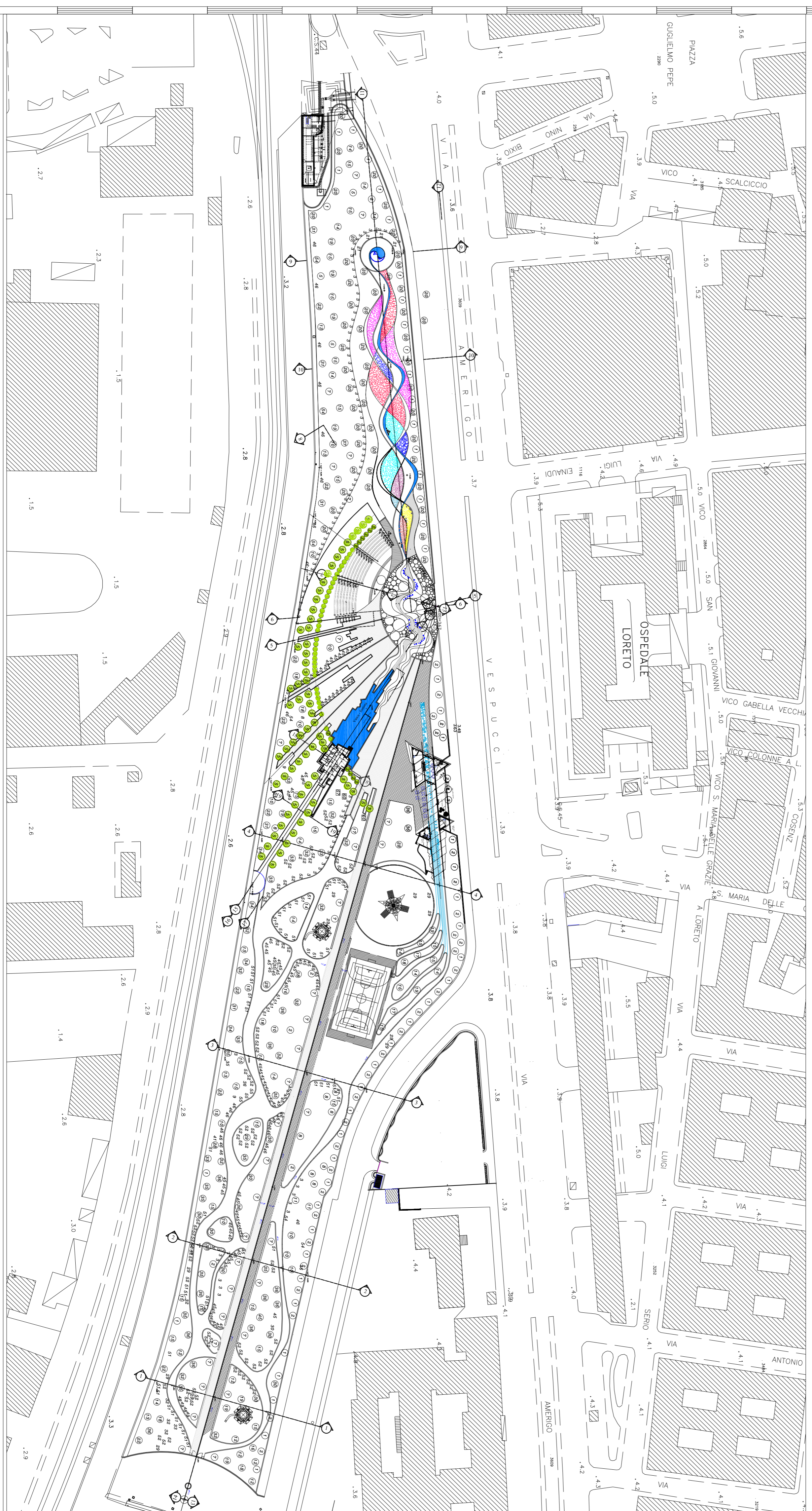
Inquadramento urbanistico 1:1000
