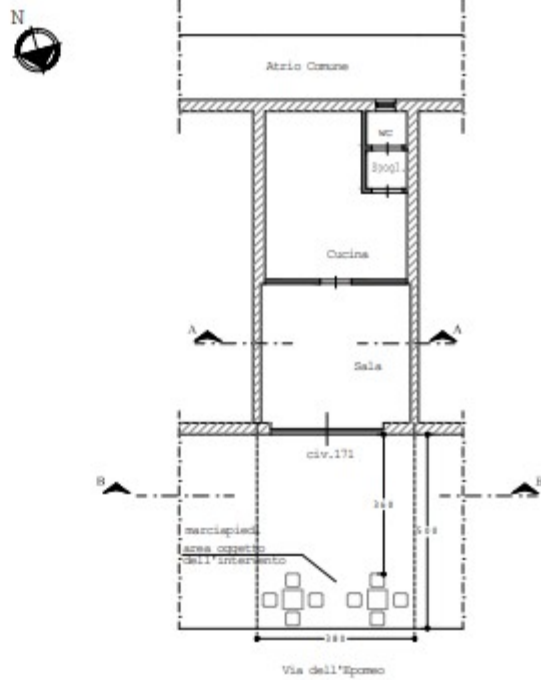
PROGETTO: Pianta scala 1:100
