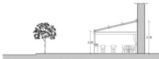
SEZIONE - PROSPETTO LATERALE - SCALA 1:100
