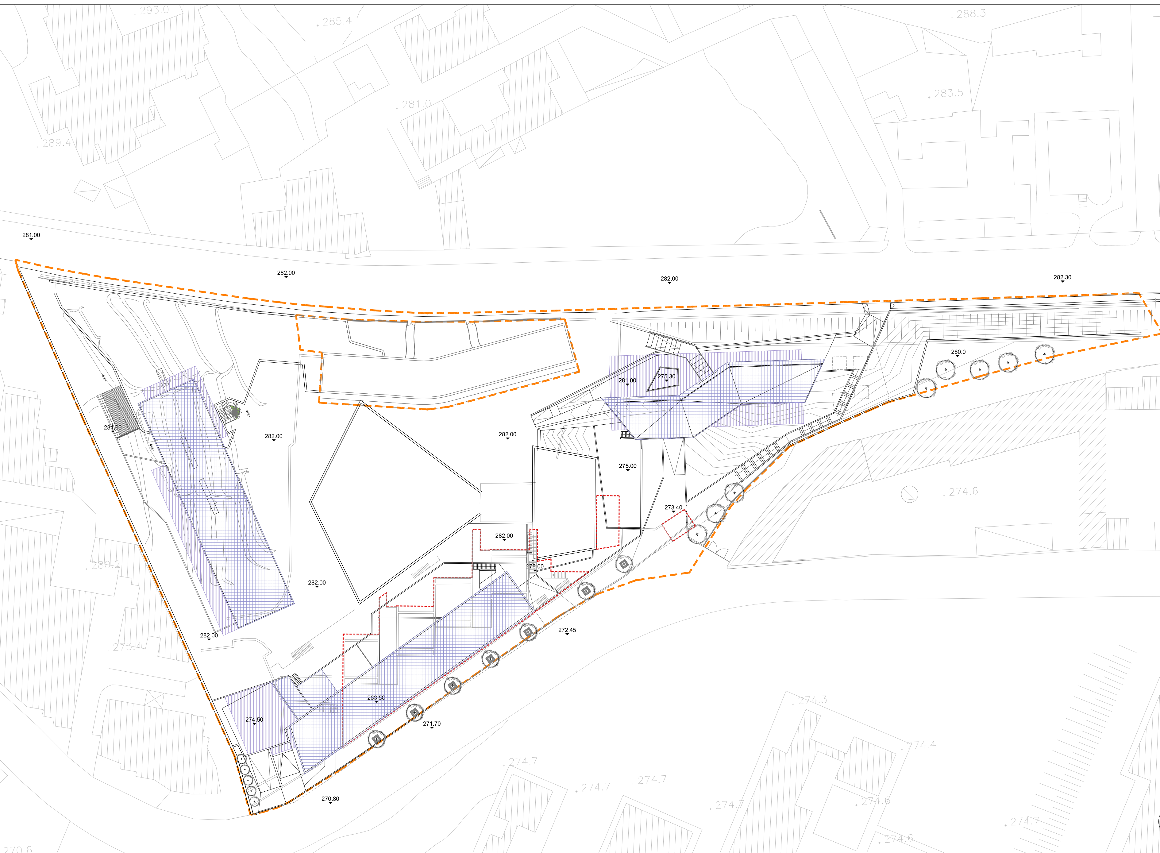
pianta delle nuove costruzioni
