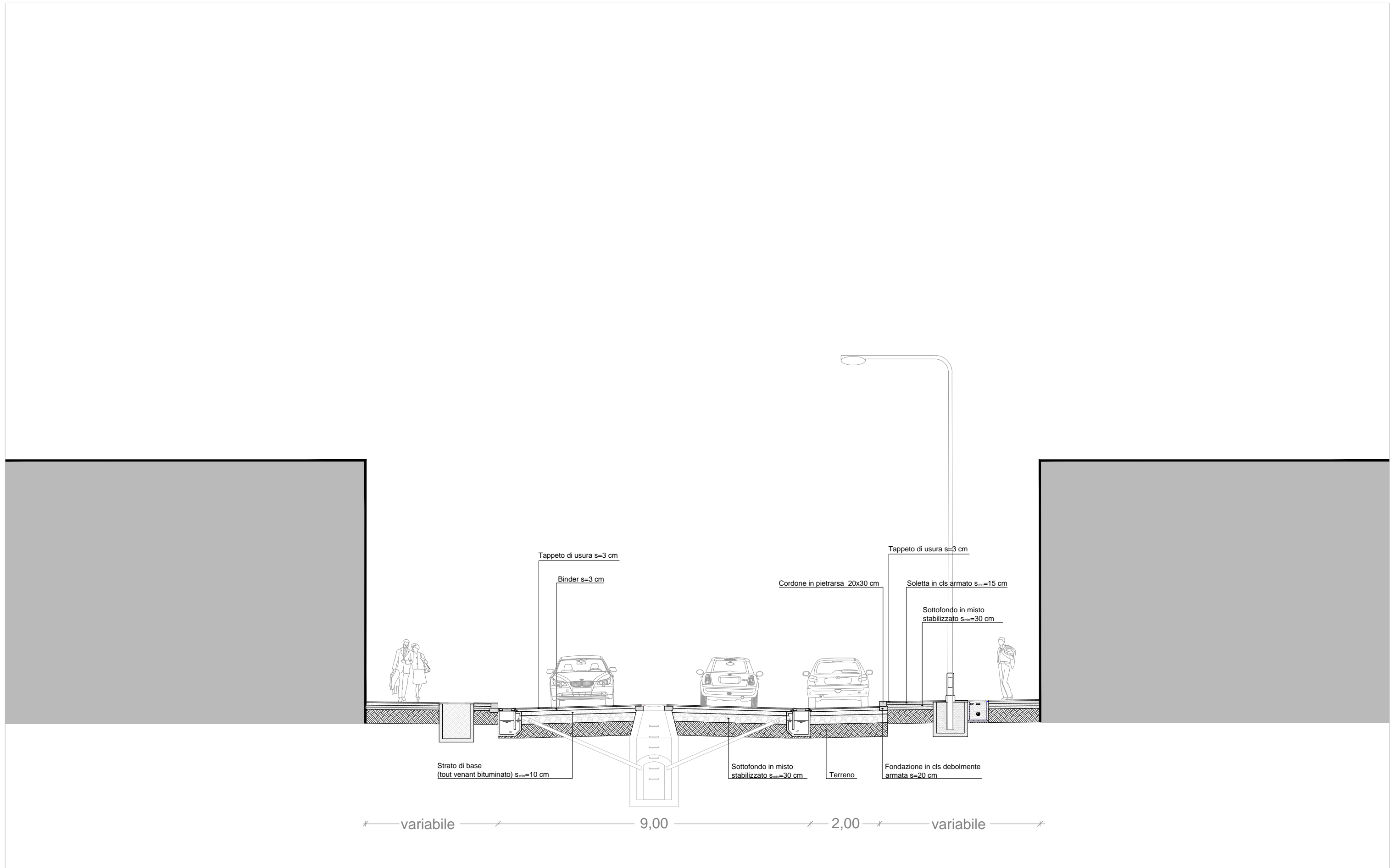
Via Nuova delle brecce - sezione tipo, scala 1:100
