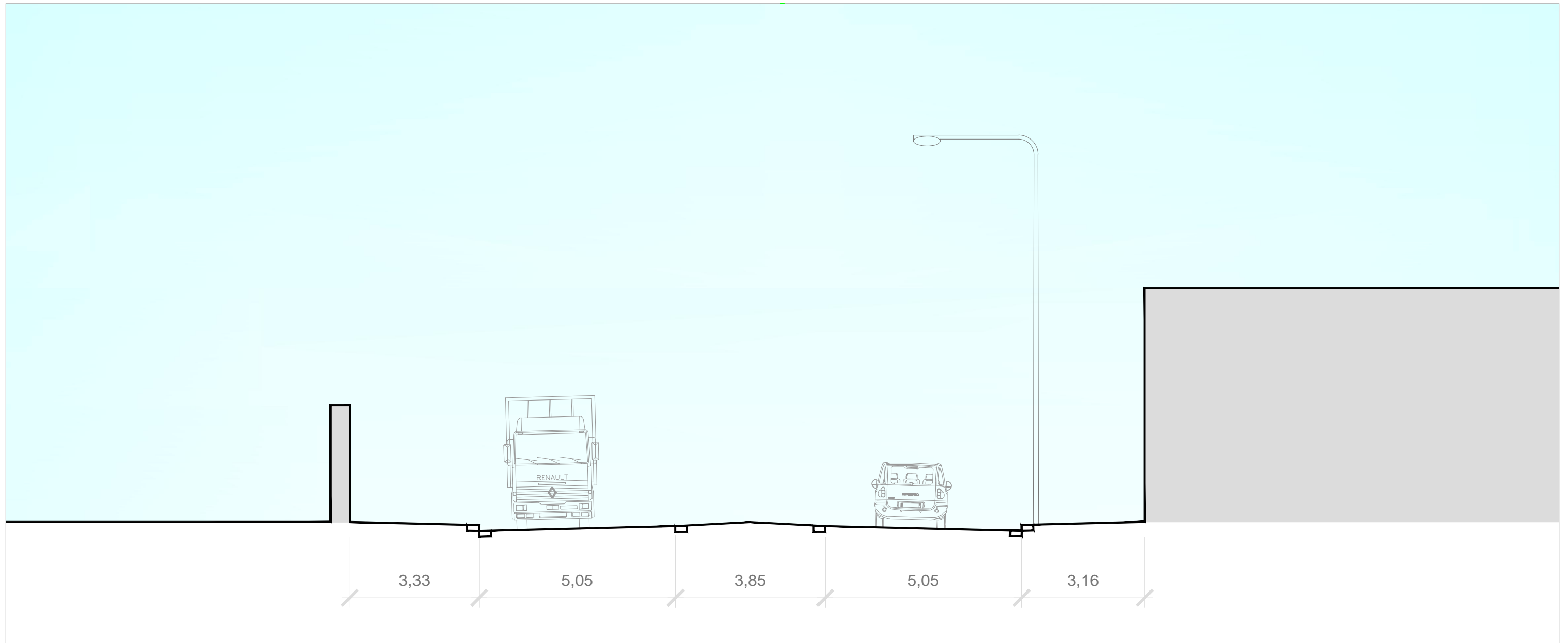
Via Nuova delle brecce, tratta via delle Industrie/fine strada - SEZ. 9, scala 1:100
