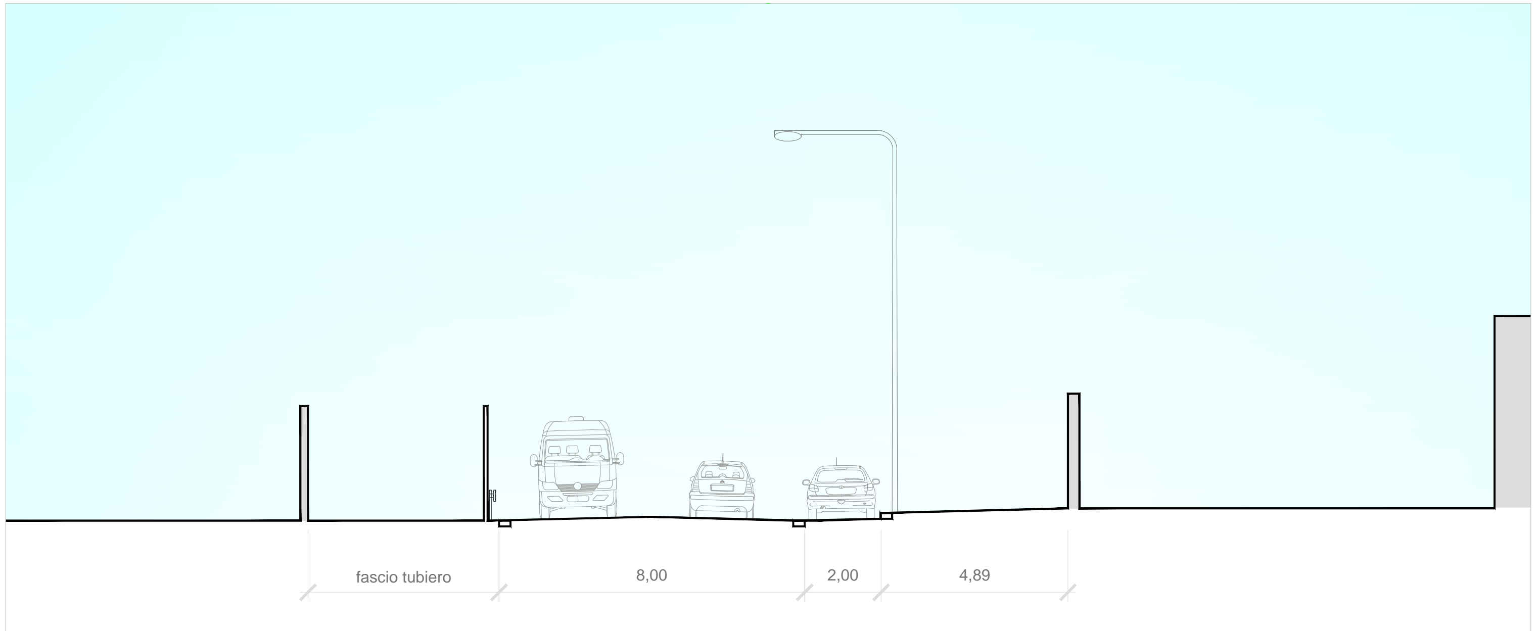
Via Nuova delle brecce, tratta via delle Industrie/fine strada - SEZ. 4, scala 1:100
