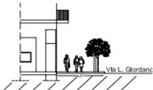
Sezione Sc:1.100 - stato di progetto
