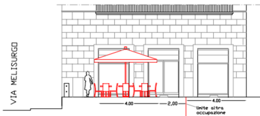
PROSPETTO/SEZIONE DI PROGETTO DELL'AREA DA OCCUPARE - SCALA 1:100
