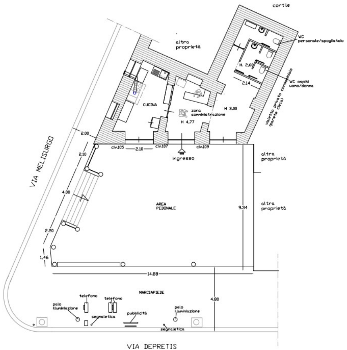
DI ANIMETRIA DI RILIEVO DELL'AREA DA OCCUPARE - SCALA
