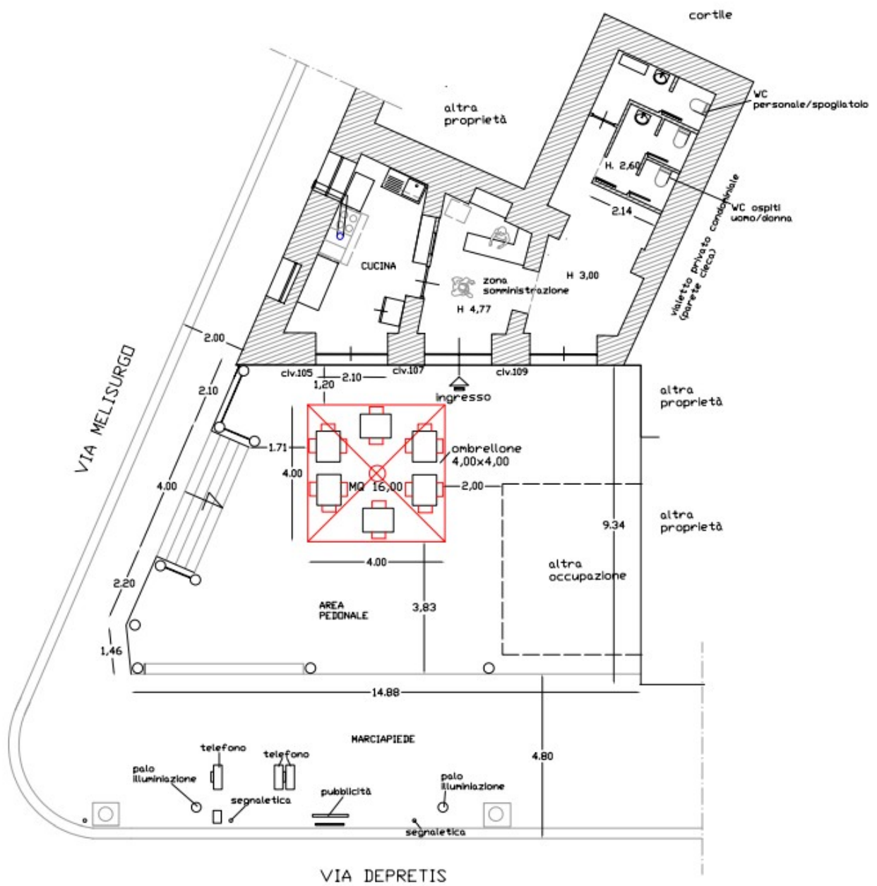
PLANIMETRIA DI PROGETTO DELL'AREA DA OCCUPARE - SCALA
