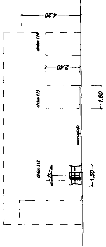
Stato di Progetto Prospetto principale
