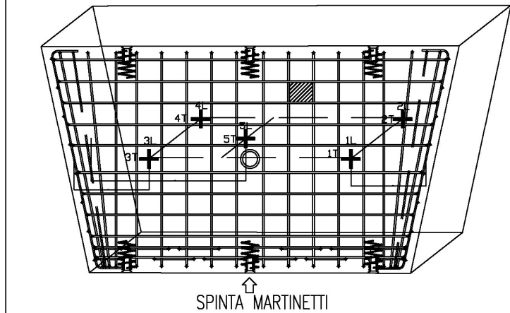
Schema concio con posizionamento barrette estensimetriche c.l.s.
