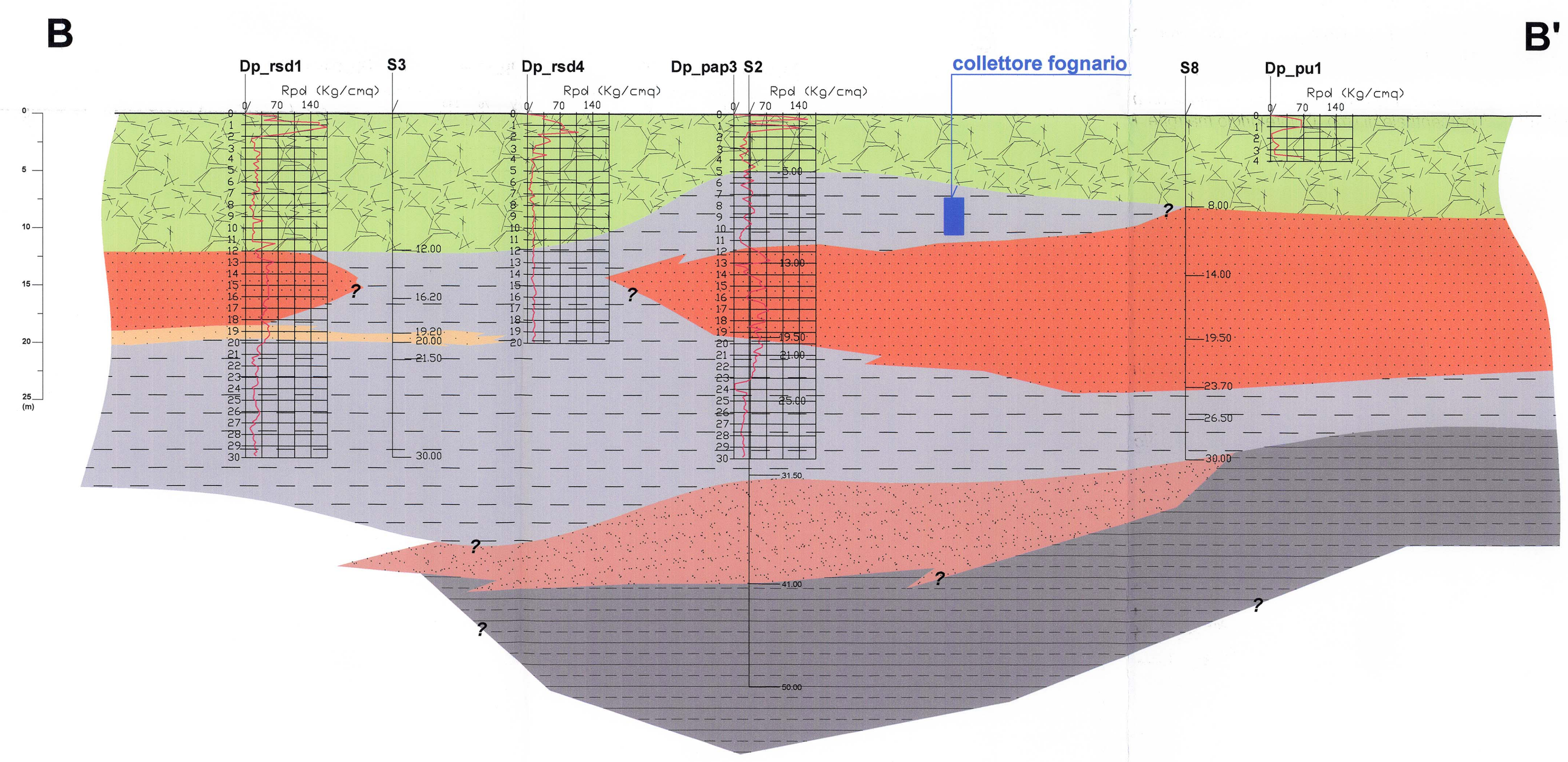
Sez: B-B'
