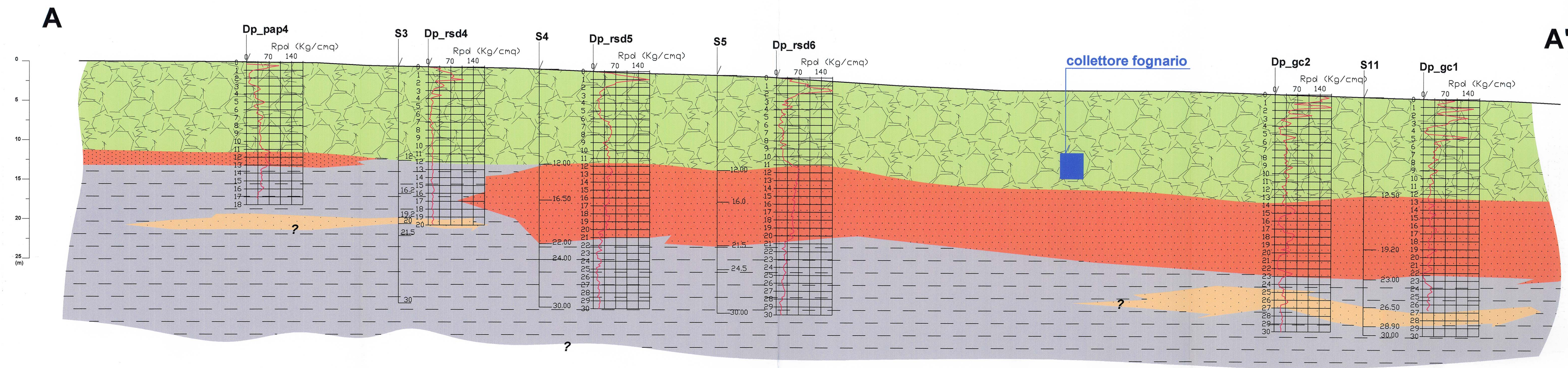
Sez: A-A'
