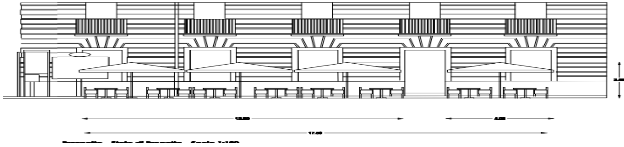
Prospetto su Via Nicolò Tommaseo - Stato di Progetto - Scala 1:100
