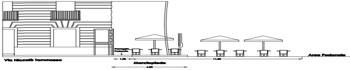
Prospetto su Via Nicolò Tommaseo - Stato di Progetto - Scala 1:100
