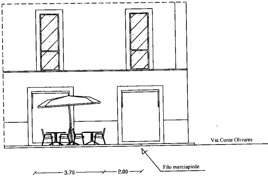
Prospetto AB - Via Conte Olivares - scala 1:100
