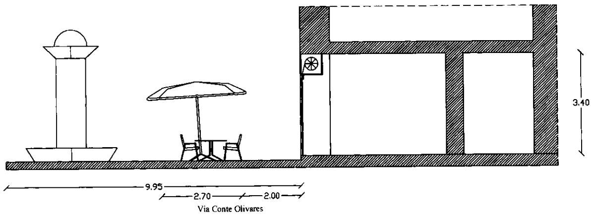
Sezione AB - scala 1:100
