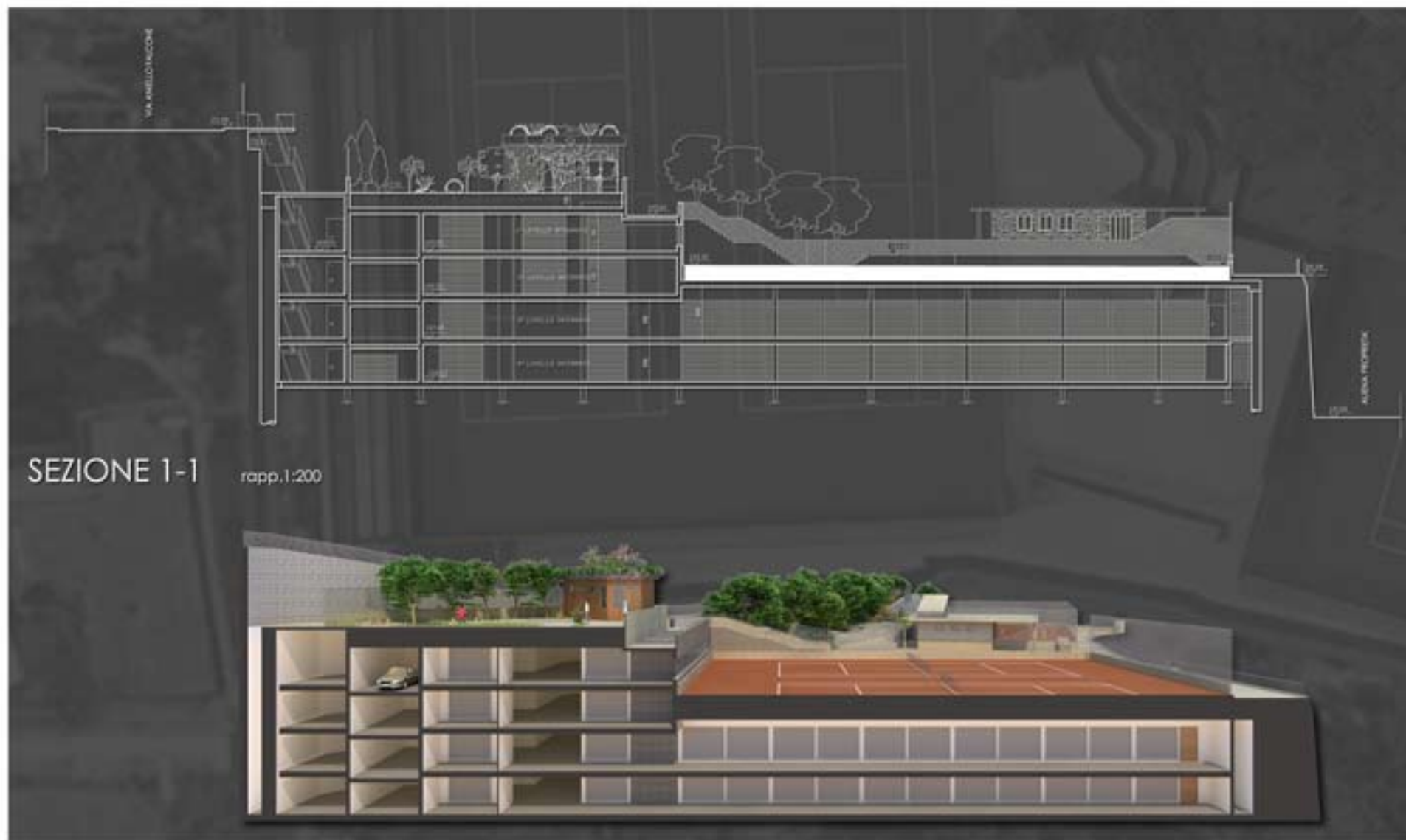
fig. 3 vista da ovest della sezione nord-sud dell'impianto finito
