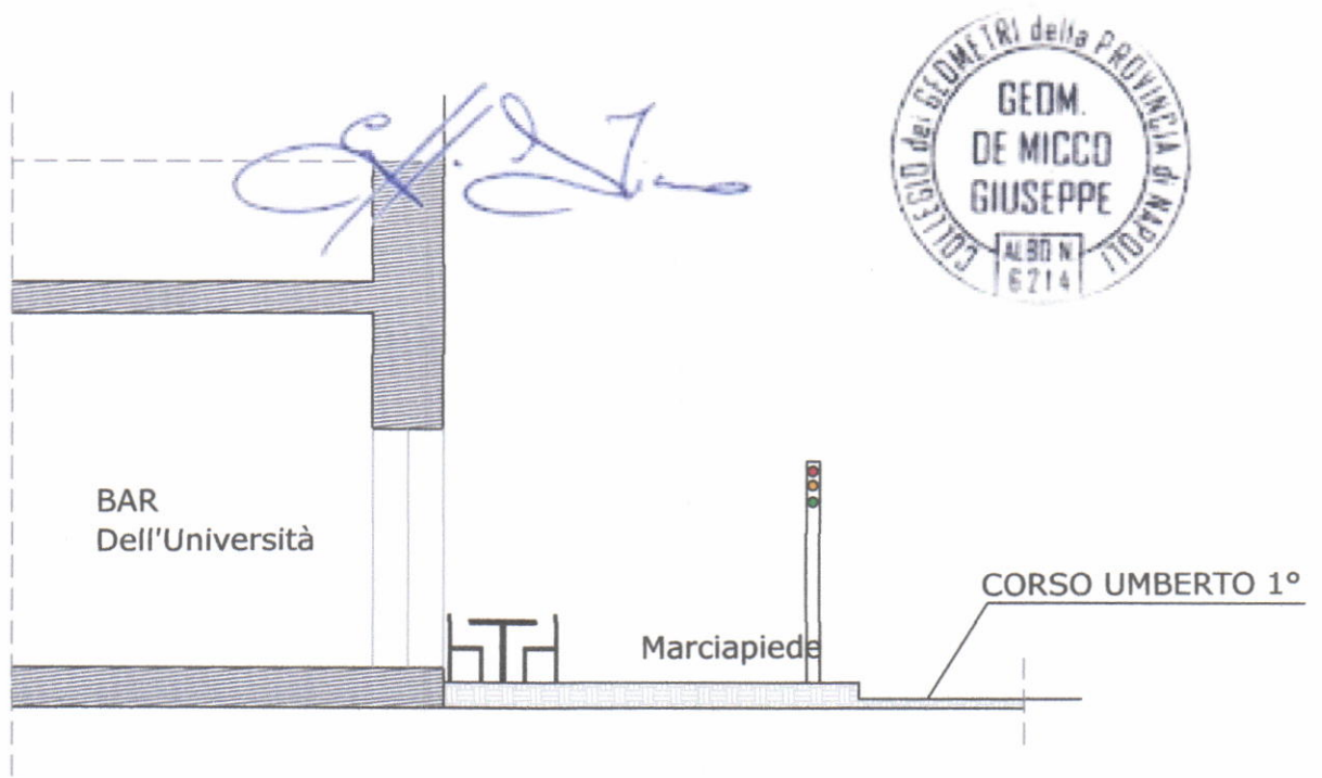
SEZIONE DI PROGETTO
