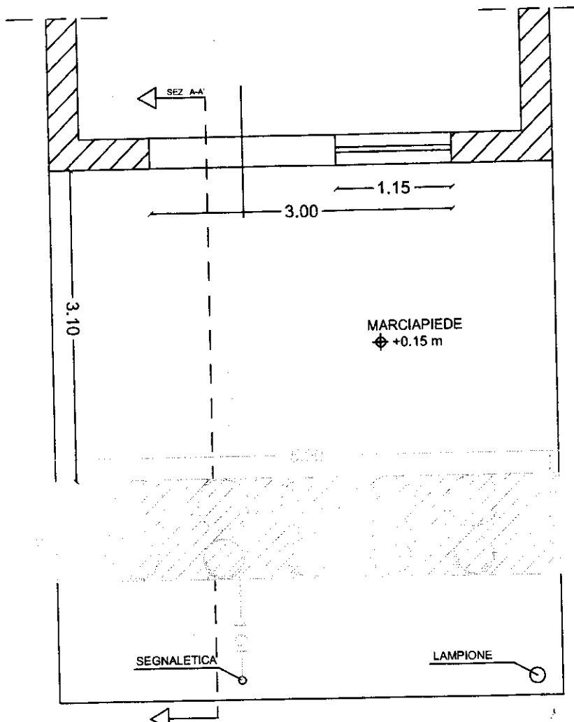
PLANIMETRIA STATO DI PROGETTO SITO IN C.SO NOVARA N°01/G SCALA 1:50
