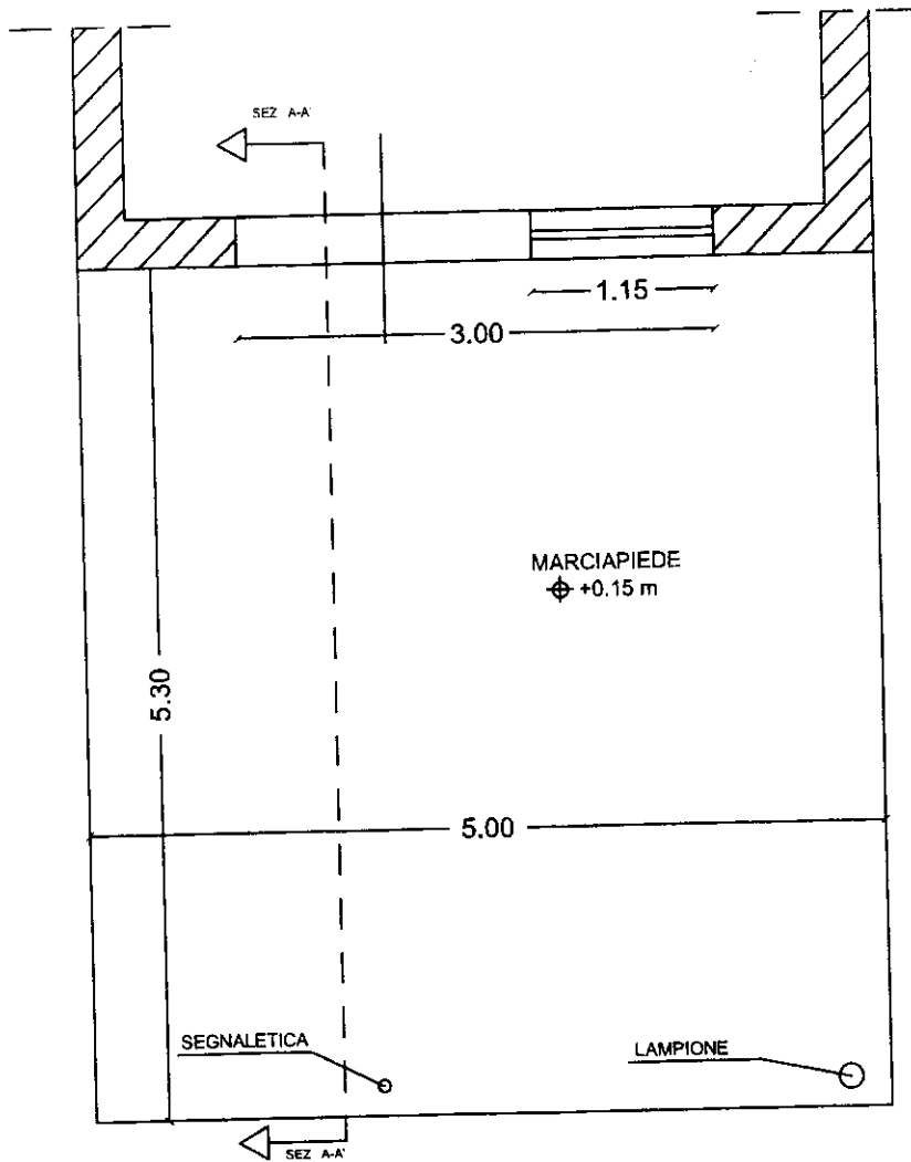
PLANIMETRIA STATO DEI LUOGHI SITO IN C.SO NOVARA N°01/G SCALA 1:50
