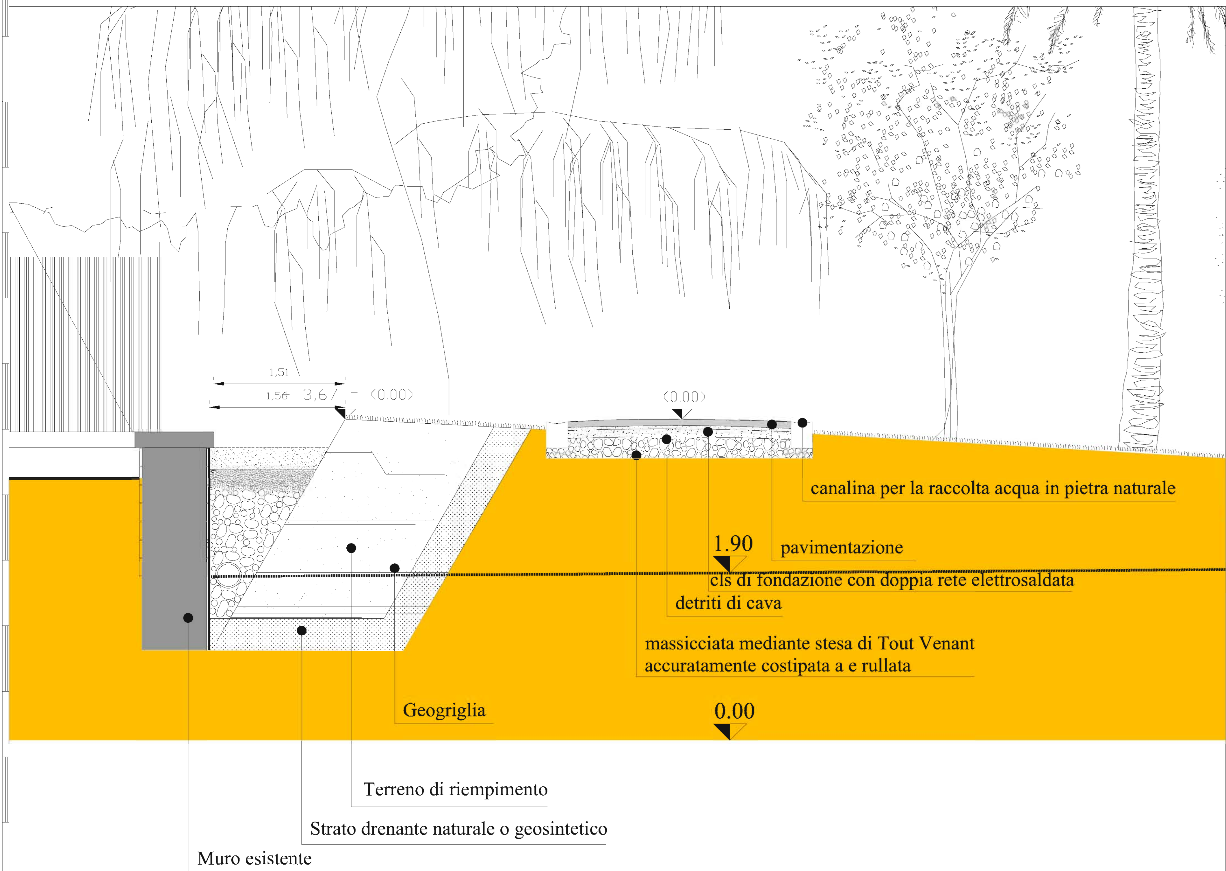
Part. A - Sez. n° 2 scala 1: 25
