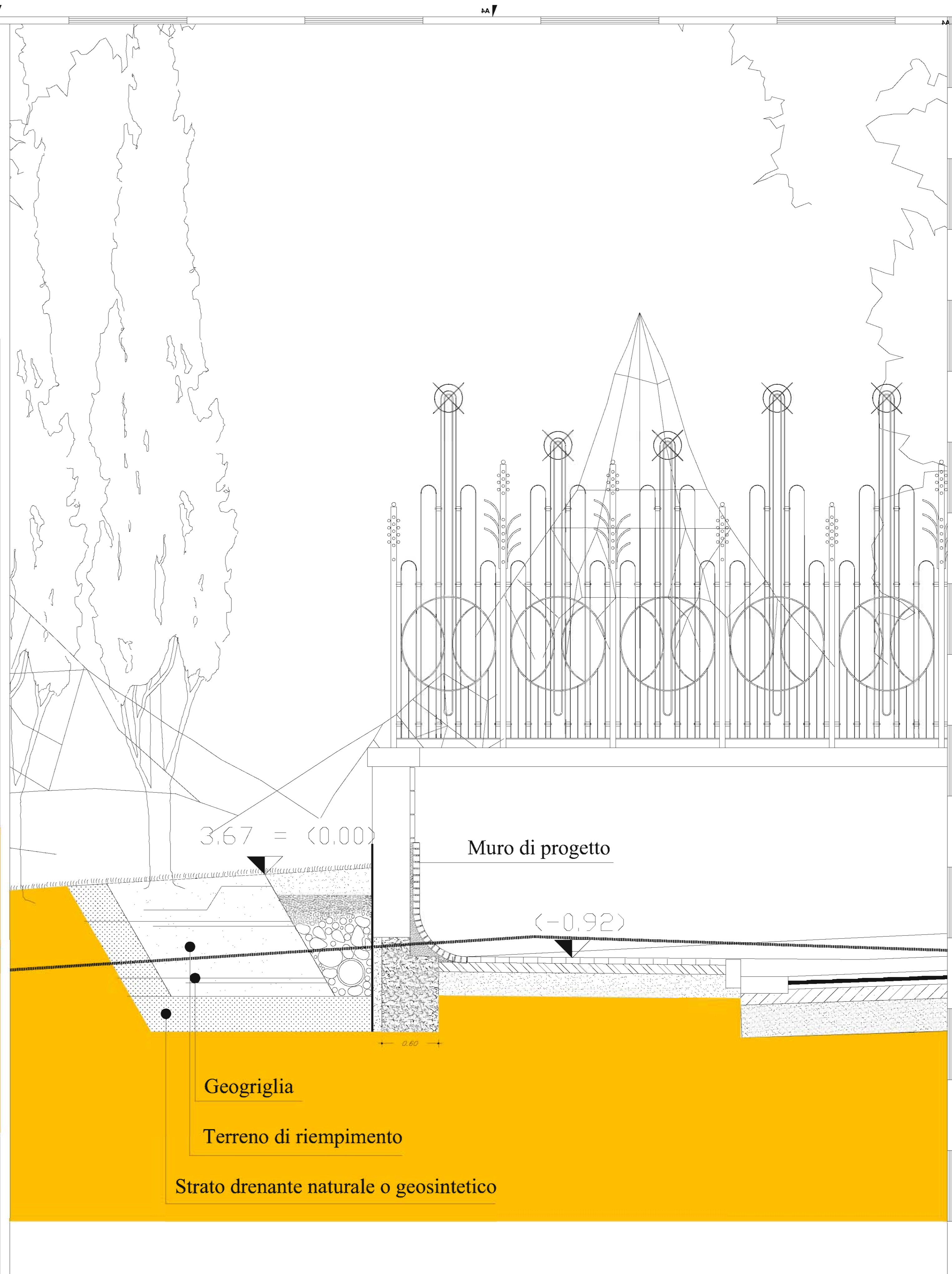
Part. B - Sez. n° 1 scala 1: 25
