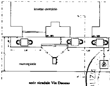
Pianta stato di progetto
