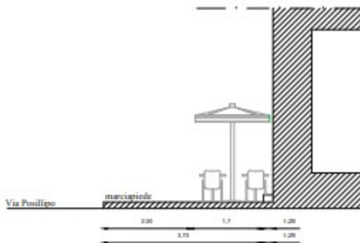
SEZIONE A - A' STATO DI PROGETTO
