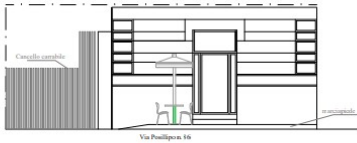
PROSPETTO STATO DI PROGETTO
