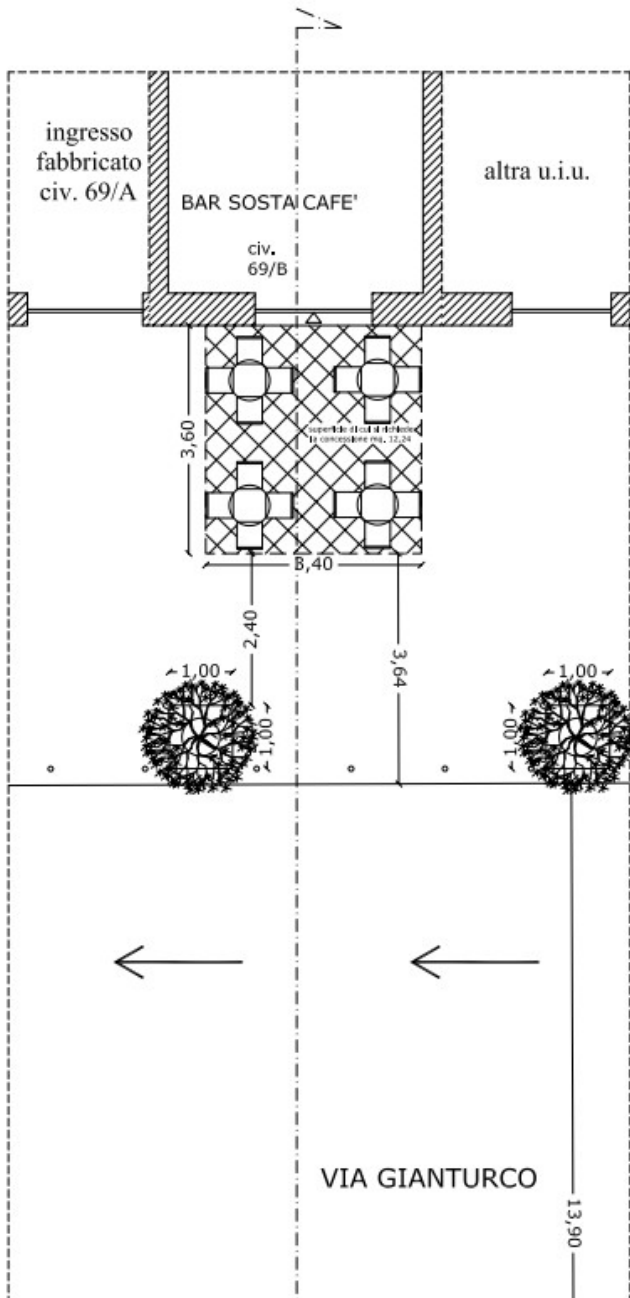
PIANTA STATO DI PROGETTO AREA ANTISTANTE L'ESERCIZIO COMMERCIALE DI CUI SI RICHIEDE LA CONCESSIONE RAPP. 1:50
