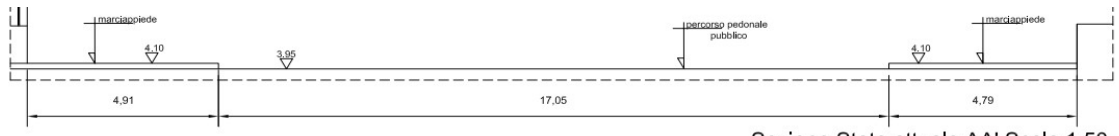
Sezione Stato attuale AA' Scala 1:50
