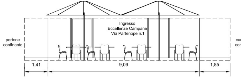
sezione BB' di Progetto scala 1:50
