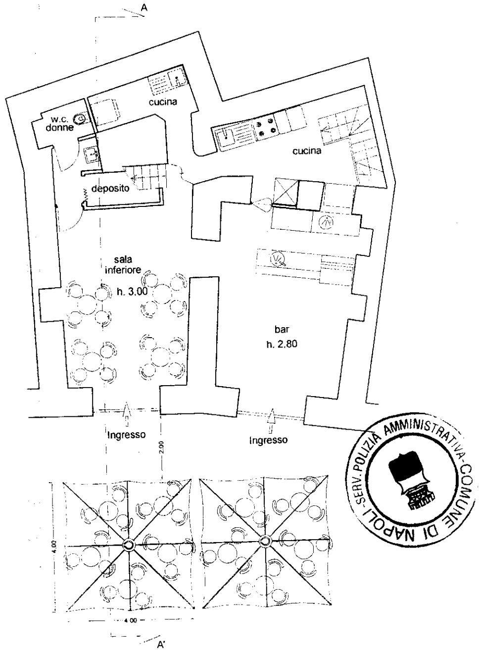
Planimetria scala 1:100
