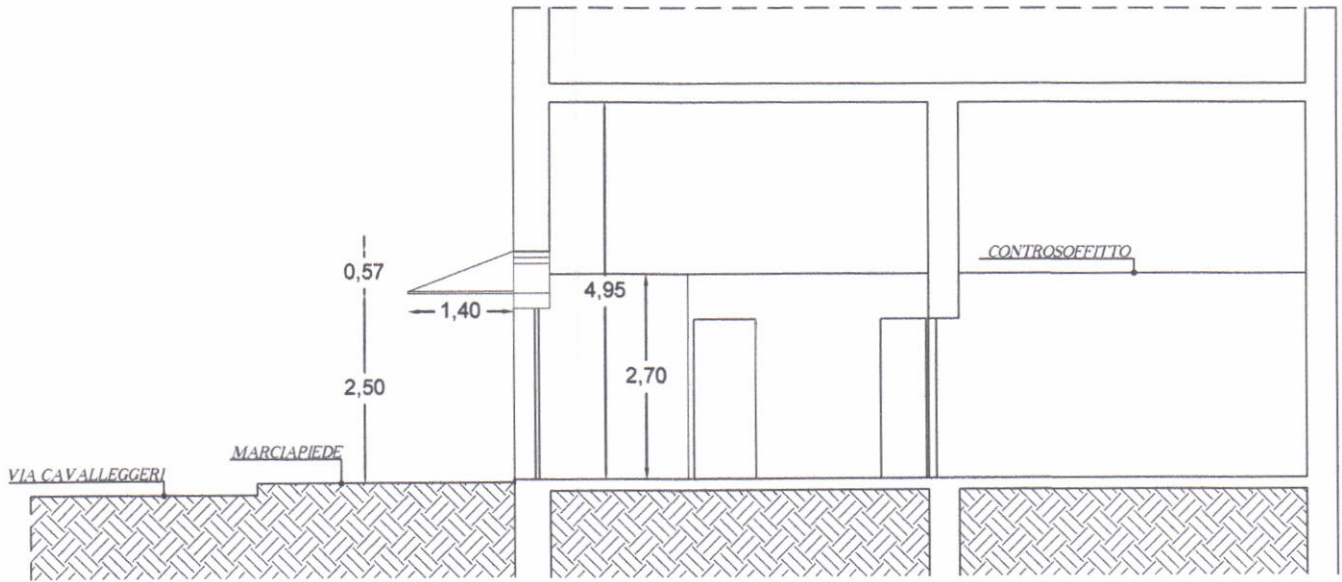
SEZIONE A-A
