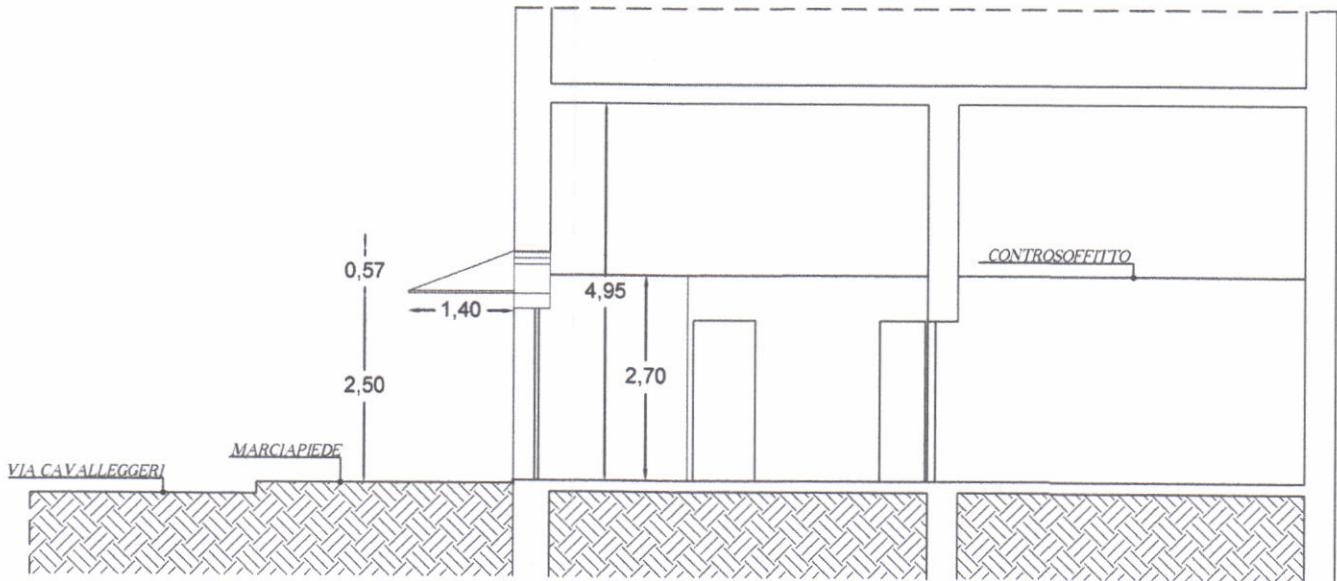
SEZIONE A-A
